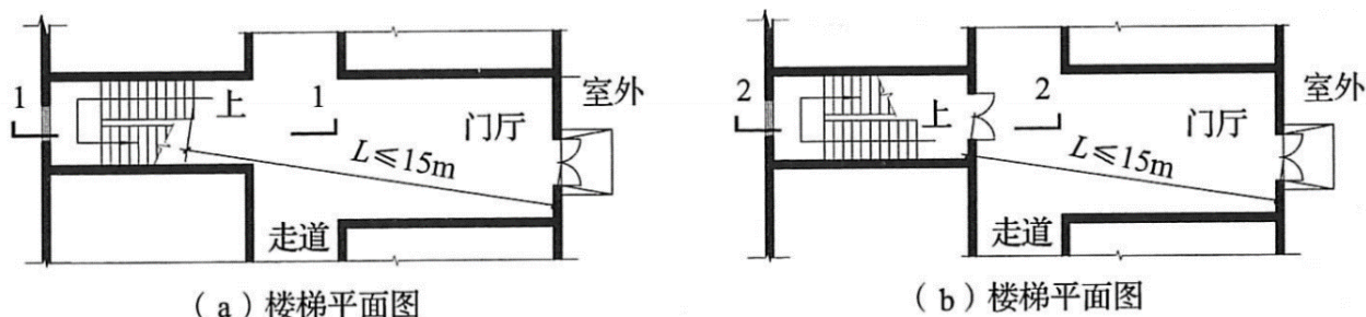
2.5.41.1 图示 疏散楼梯首层门厅示意图
