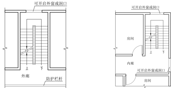
2.5.23 图示一 敞开楼梯间平面示意图
