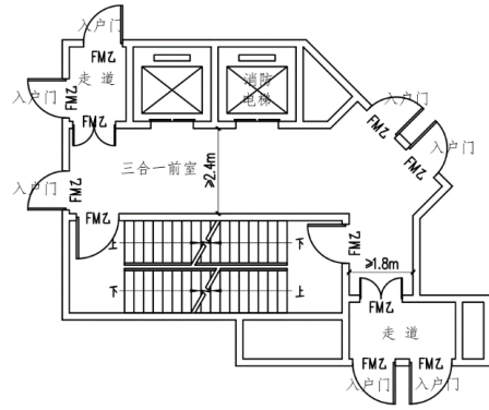
2. 5. 62 图示二十三 (✗) 注释：单元总户数不应超过 6 户。
