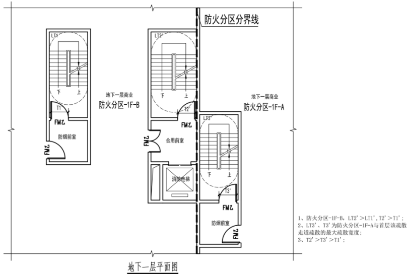
地下一层平面图 地下二层功能为车库及设备用房等
