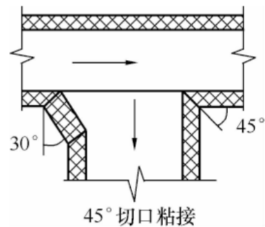
图 4.5.6 主风管上直接开口连接支风管方式
