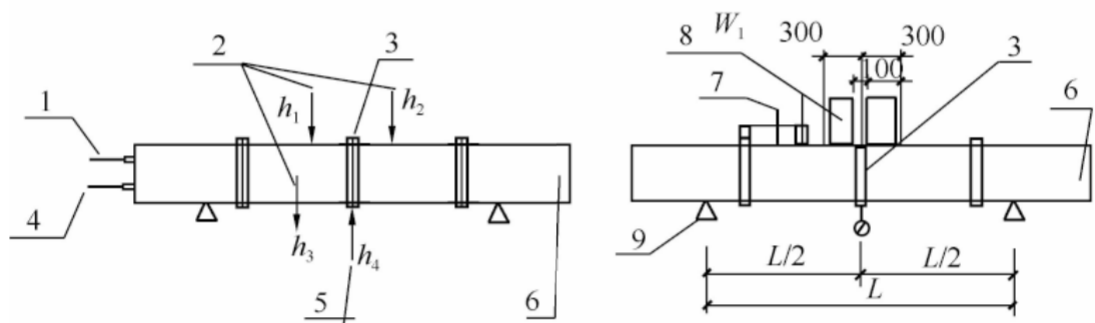
图 A. 4.1 风管测试装置图
