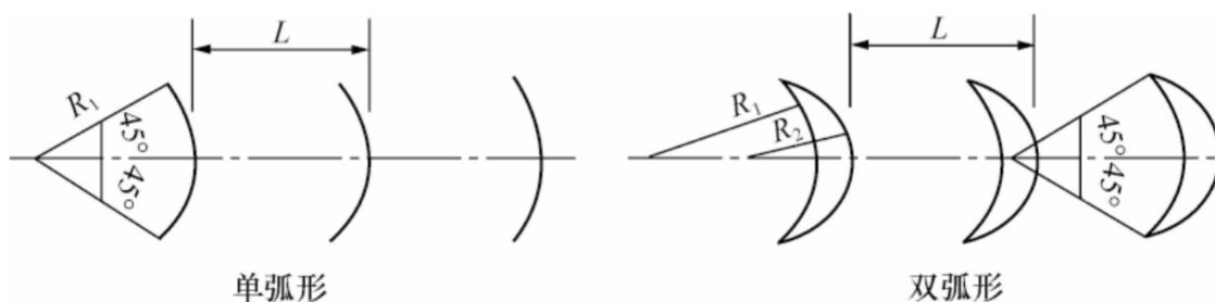
图 3.11.2-2 导流片形式
