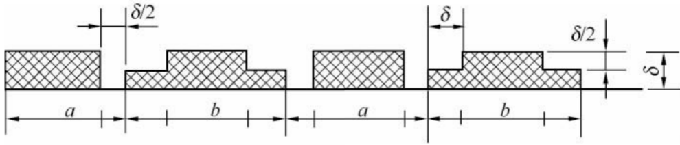
图 3.6.2-2 玻璃纤维复合板风管 90°梯形槽口
