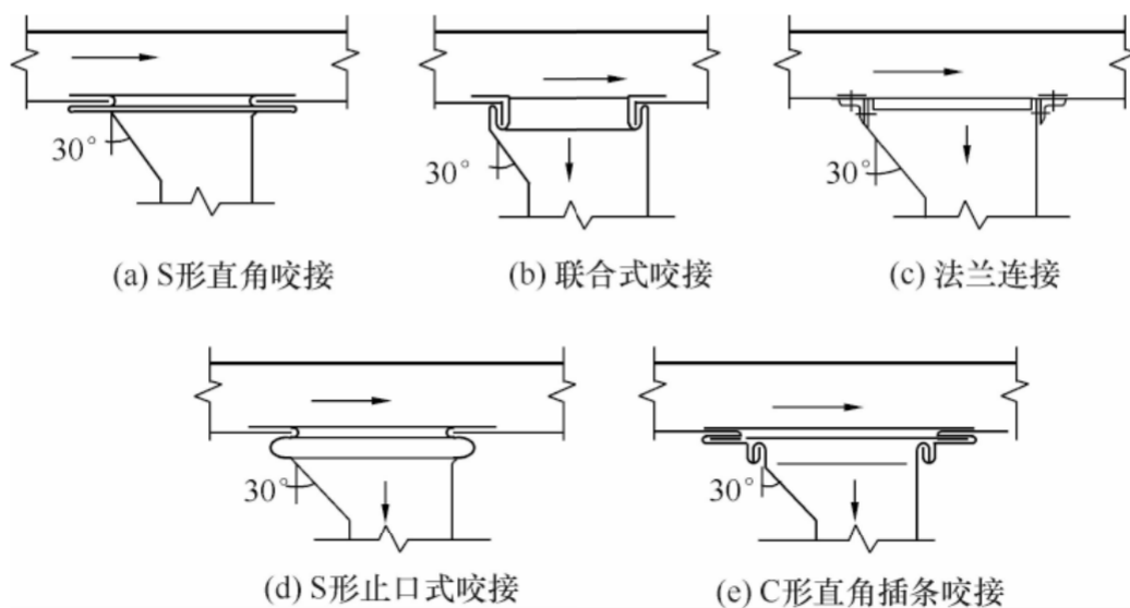
图 4.4.7 支风管与主风管连接方式
