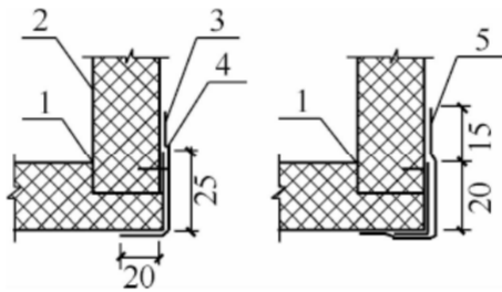
图 3.6.2-3 风管制作直角成型形式图
