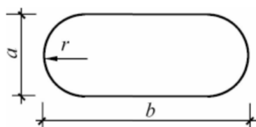
图 2.0.13 扁圆形风管表示方法
