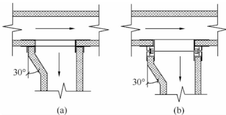
图 4.3.8 主风管与支风管 90^\circ 连接示意图
