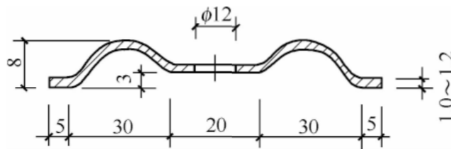
图 3.6.2-4 波纹槽形加固件
