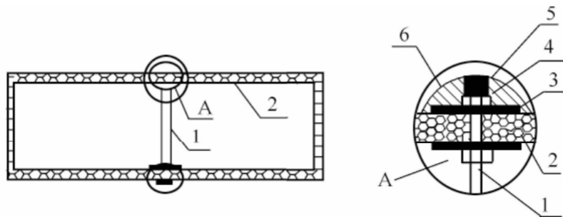
图 3.6.4-8 隔热风管内支撑加固示意图
