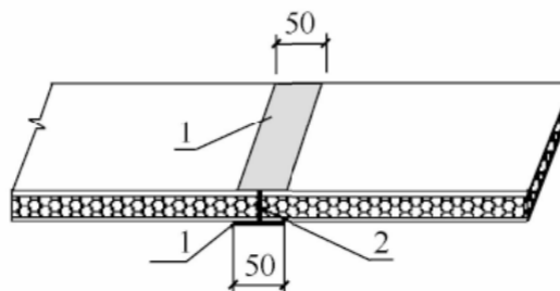
图 3.6.4-3 复合板拼接方法示意图
