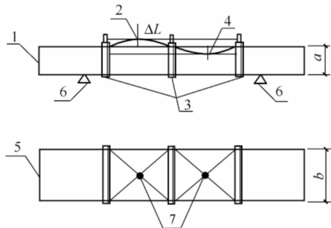
图 A. 5. 2 管壁变形量试验图
