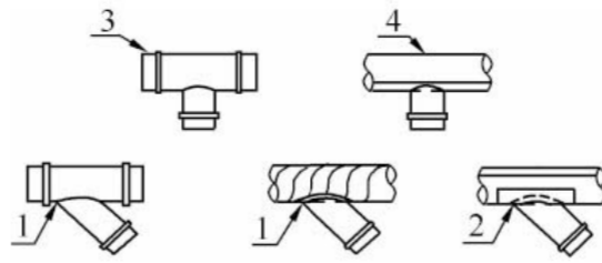
图 3.11.5 三通连接形式
