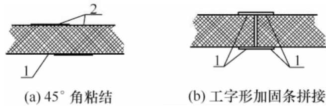
图 3.6.1-1 风管板材拼接方式
