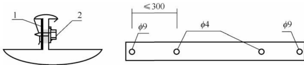
图 4. 4. 3 薄钢板法兰板条加固示意图
