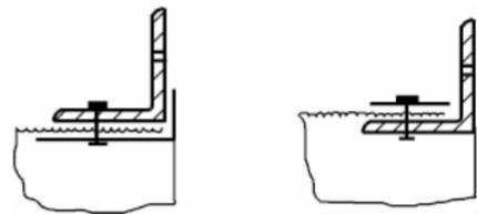
图 4.7.3 柔性风管与角钢法兰的连接
