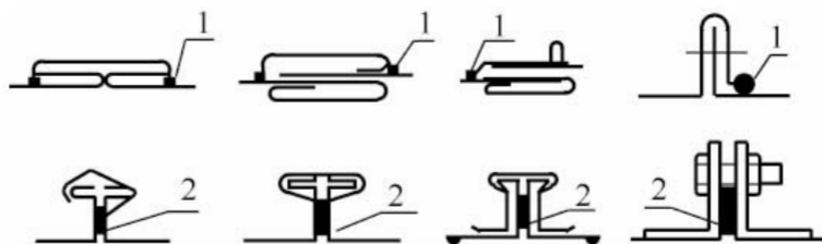
图 4.3.5-1 矩形风管管段连接的密封
