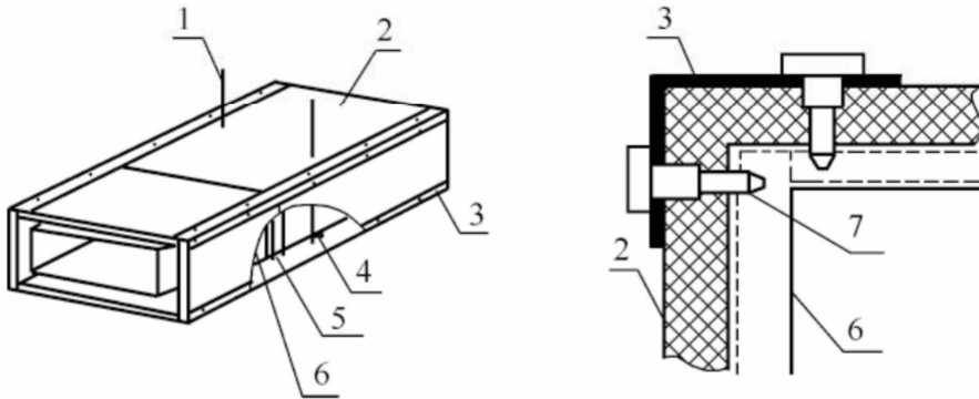
图 4.4.8 金属风管外敷防火板及角部连接图
