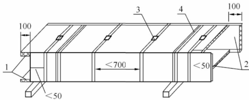
图 3.6.4-7 风管捆扎示意图
