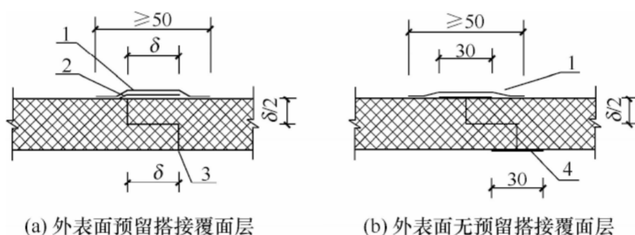
图 3.6.2-1 玻璃纤维复合板拼接
