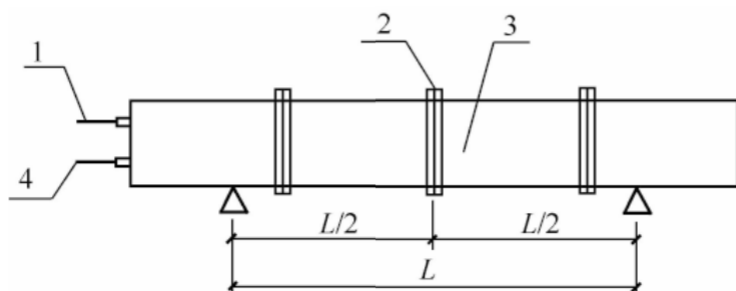
图 A.3.1 试验用风管
