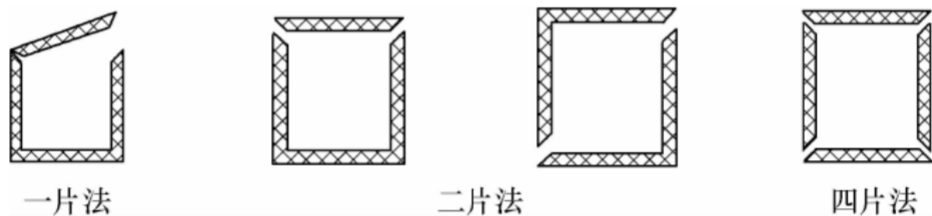
图 3.6.1-2 矩形风管 45°角组合方式
