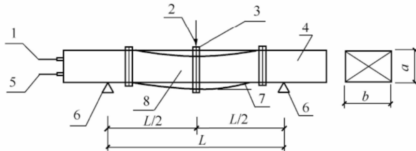
图 A. 5. 1 挠度变形量及漏风量测试图
