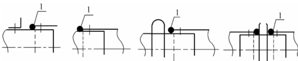
图 4.3.5-2 圆形风管管段连接的密封
