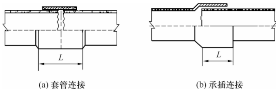
图 4.5.5 硬聚氯乙烯、聚丙烯（PP）风管连接
