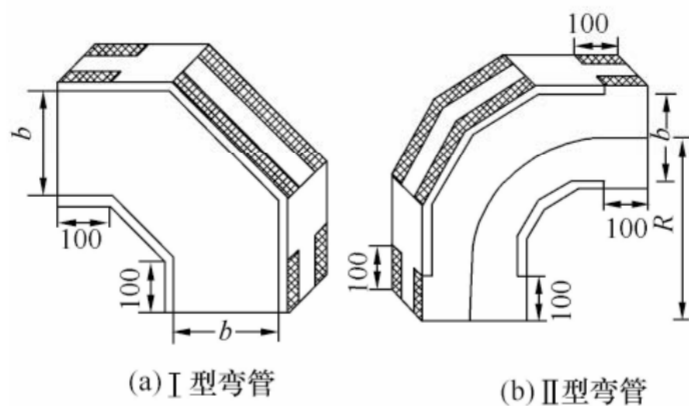
图 3.6.4-4 90°弯管放样下料示意图
