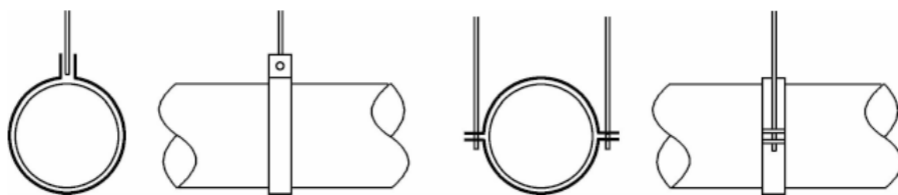
图 4.2.14 柔性风管卡箍安装
