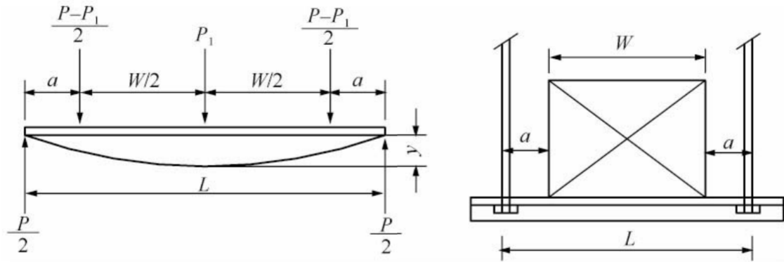
图 4.2.3 吊架载荷分布图
