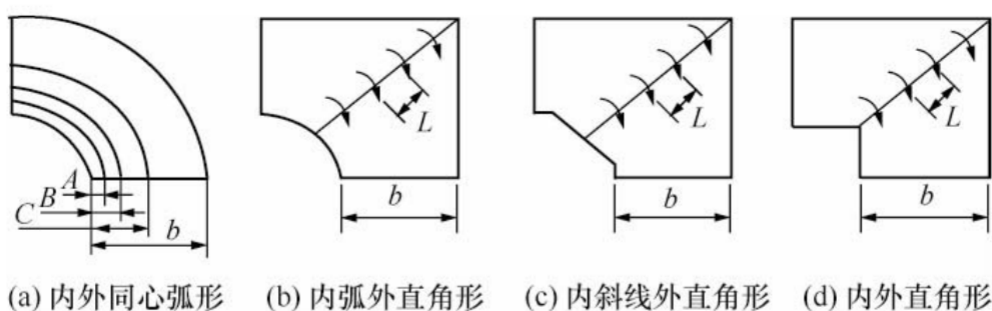
图 3.11.2-1 矩形弯管示意图
