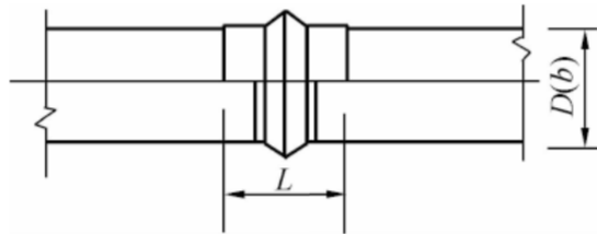
图 4.5.8 风管软接头示意图
