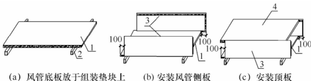
图 3.6.4-6 风管组装示意图
