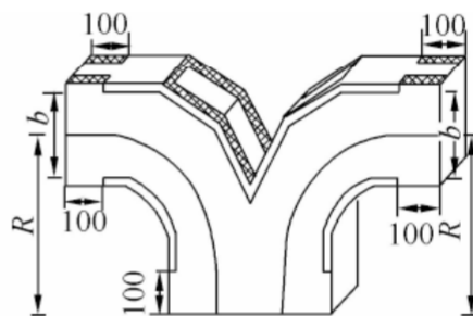
图 3.6.4-5 三通放样下料示意图
