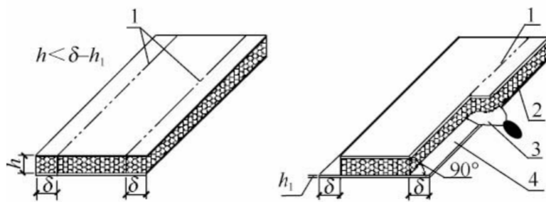
图 3.6.4-1 风管侧板阶梯线切割示意图
