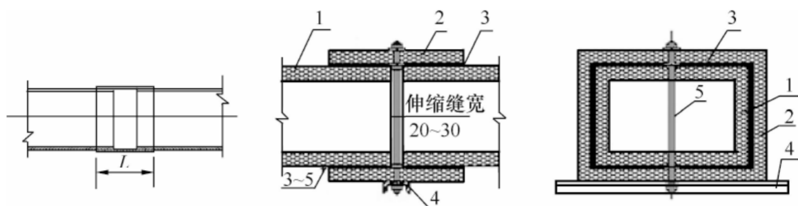
图 3.6.4-9 伸缩节构造示意图
