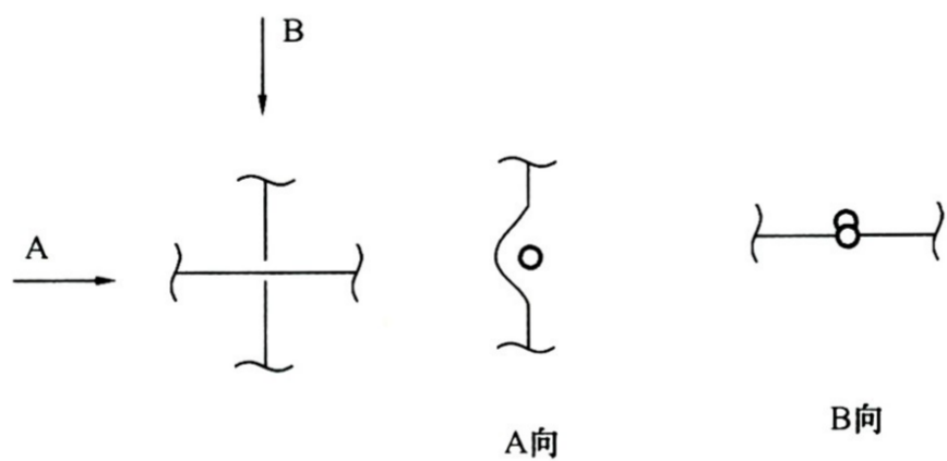
图 4.6.10 管道跨越的画法
