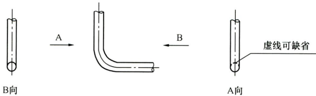
图 4.6.2 双线管道转向的画法
