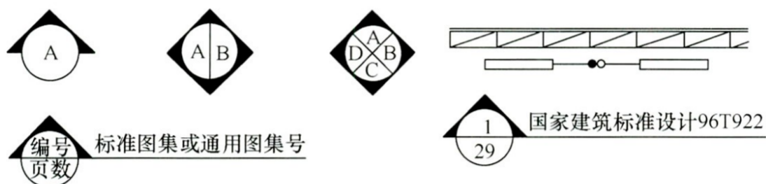
图 4.2.11 内视符号画法
