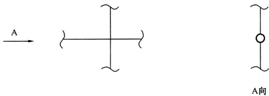
图 4.6.9 管道交叉的画法
