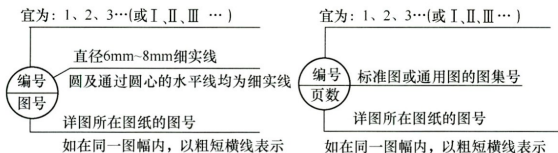
图 4.2.10 索引符号的画法
