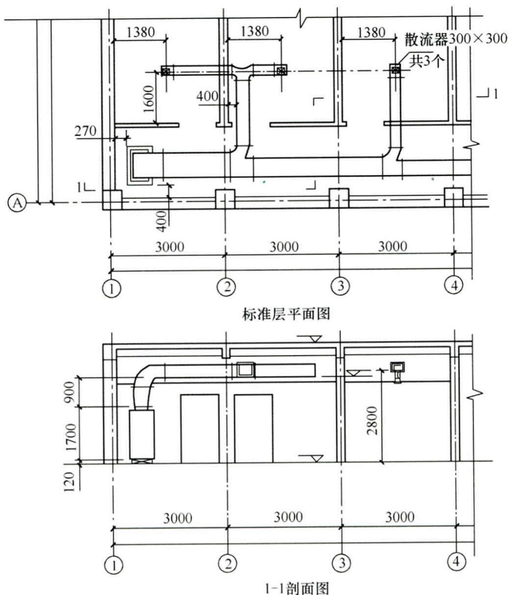
图 4.2.3 平、剖面示例
