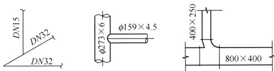
图 4.5.12 管道截面尺寸的画法
