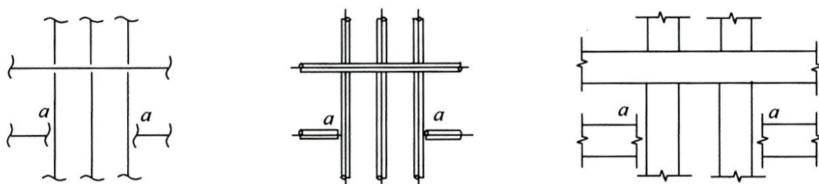
图 4.6.7 管道断开的画法
