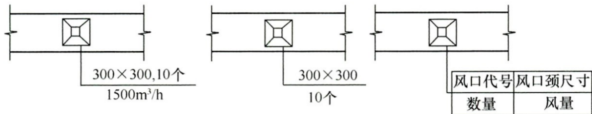
图 4.5.15 风口、散流器的表示方法
