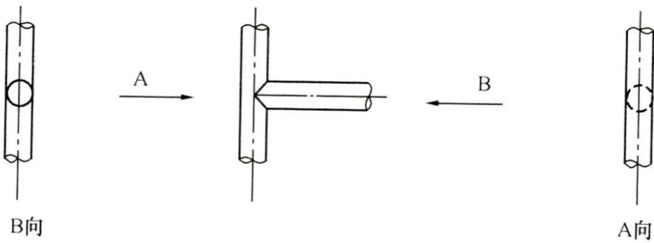
图 4.6.4 双线管道分支的画法
