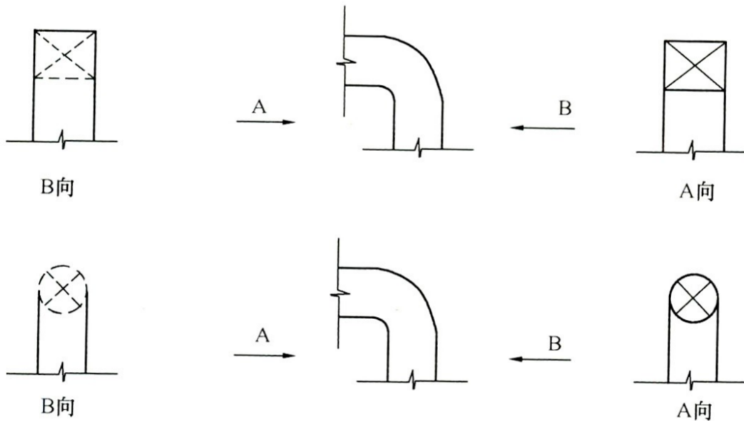
图 4.6.5 送风管转向的画法
