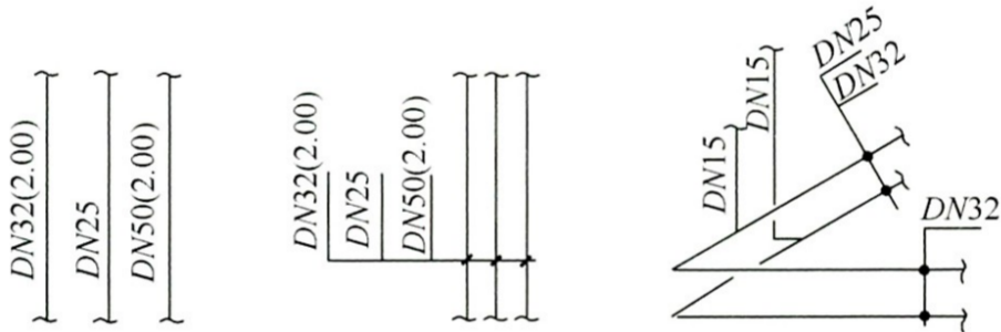
图 4.5.13 管径（压力）的标注位置示例
