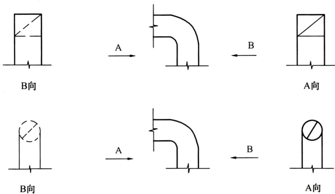
图 4.6.6 回风管转向的画法
