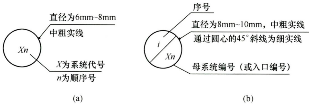
图 4.4.3 系统代号、编号的画法
