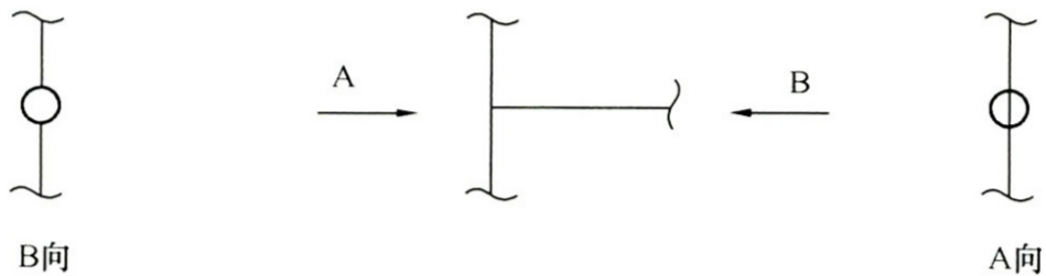
图 4.6.3 单线管道分支的画法
