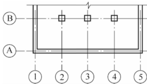
图 8.0.3 定位轴线的编号顺序
