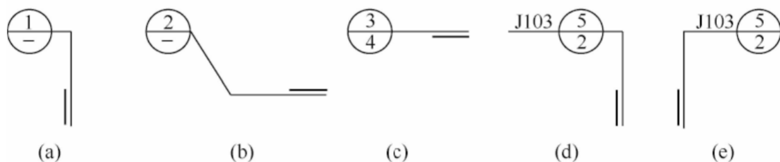
图 7.1.4-3 用于索引剖视详图的索引符号
