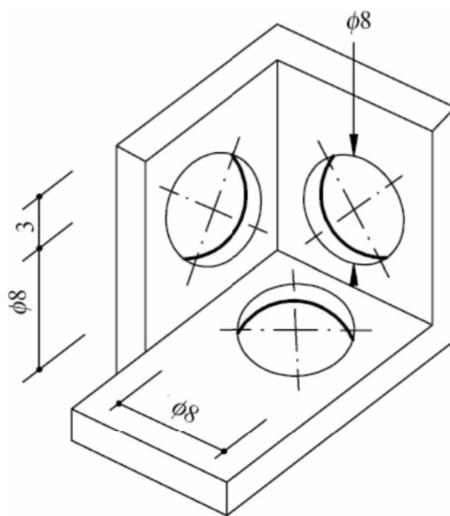
图 10.5.5 轴测图圆直径标注方法
