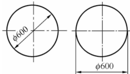
图 11.4.4 圆直径的标注方法
