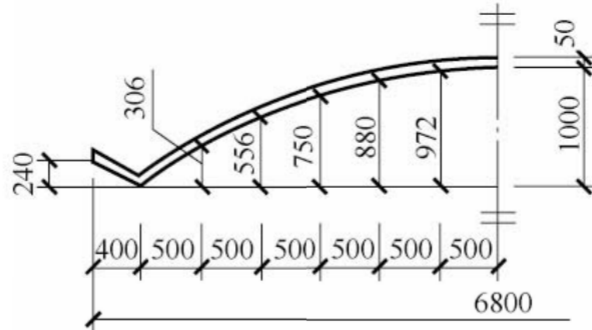
图 11.6.4 坐标法标注曲线尺寸
