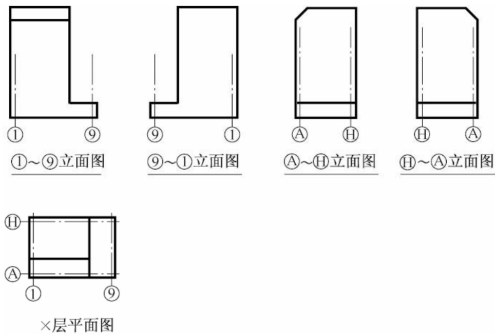
图 10.2.1 视图布置
