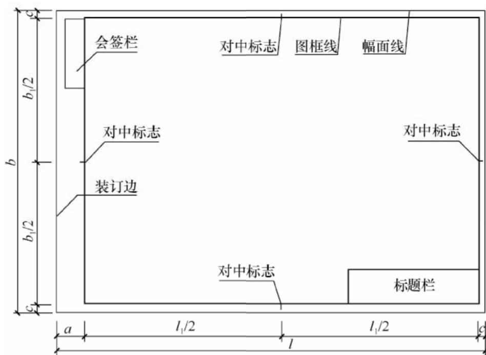
图 3.2.1-3 A0~A1 横式幅面 (三)
