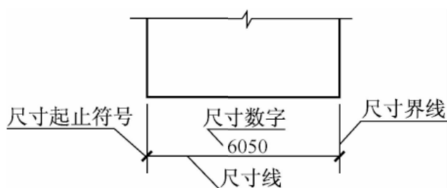
图 11.1.1 尺寸的组成
