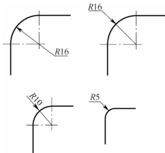
图 11.4.2 小圆弧半径的标注方法
