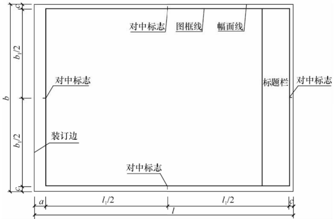
图 3.2.1-1 A0~A3 横式幅面 (一)
