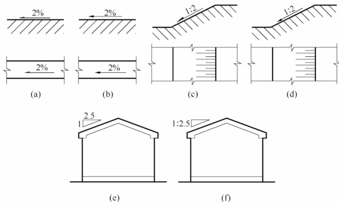
图 11.6.3 坡度标注方法
