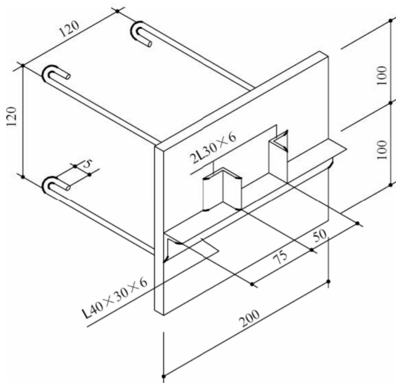
图 10.5.4 轴测图线性尺寸的标注方法
