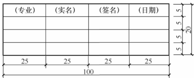
图 3. 2. 2-5 会签栏
