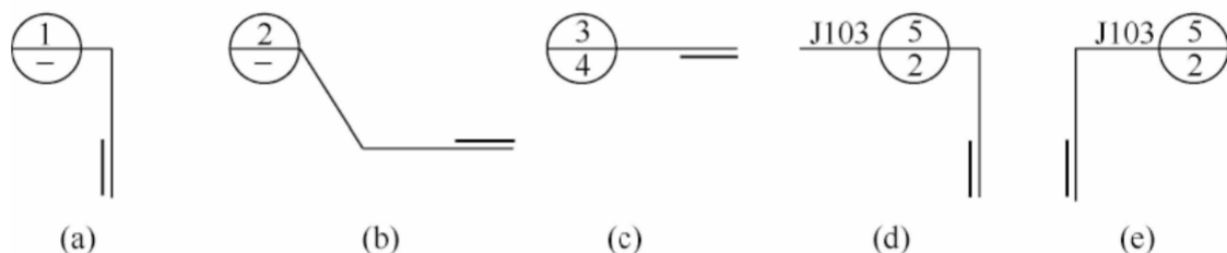
图 7.2.2 用于索引剖视详图的索引符号
