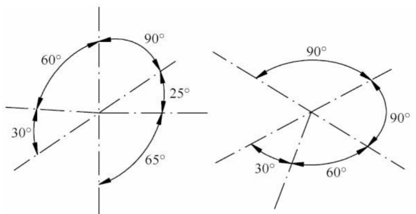
图 10.5.6 轴测图角度的标注方法
