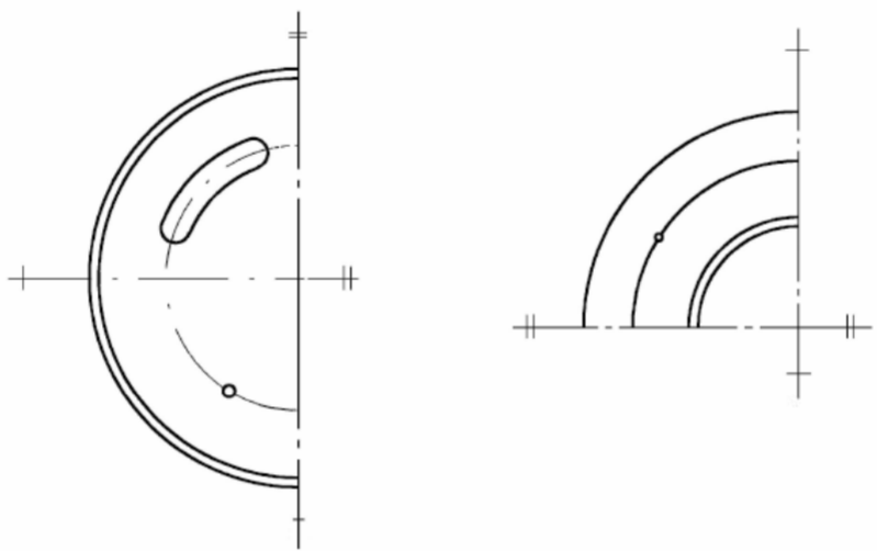
图 10.4.1-1 画出对称符号
