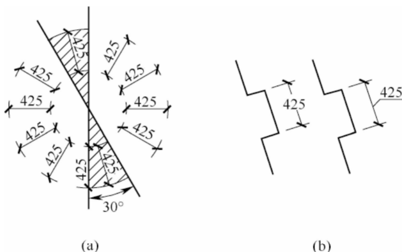
图 11.2.3 尺寸数字的注写方向
