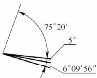
图 11.5.1 角度标注方法
