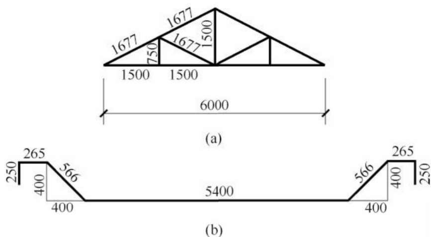
图 11.7.1 单线图尺寸标注方法
