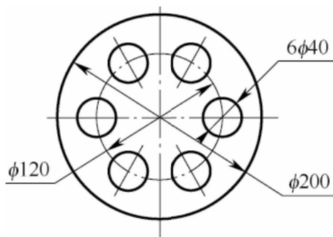
图 11.7.3 相同要素尺寸标注方法
