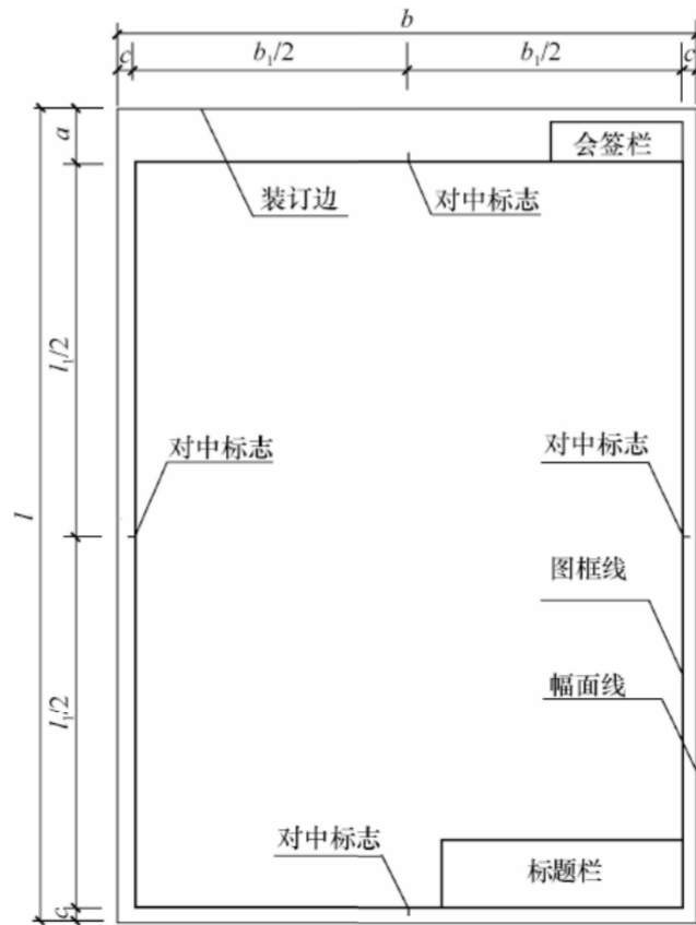
图 3.2.1-6 A0~A2 立式幅面 (三)
