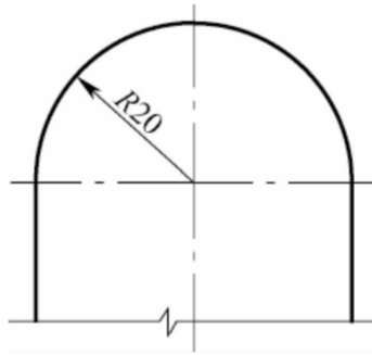
图 11.4.1 半径标注方法
