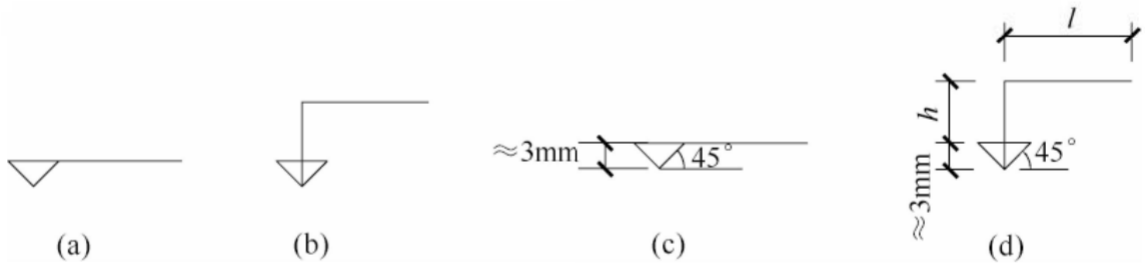
图 11.8.1 标高符号
