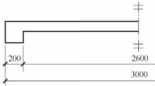
图 11.7.4 对称构件尺寸标注方法
