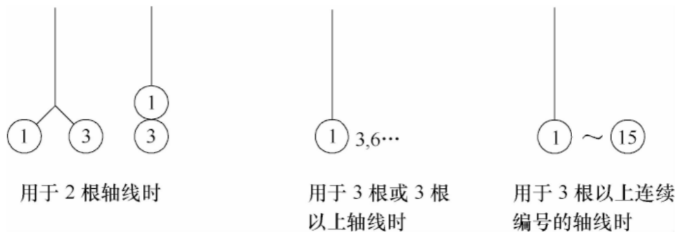
图 8.0.7 详图的轴线编号
