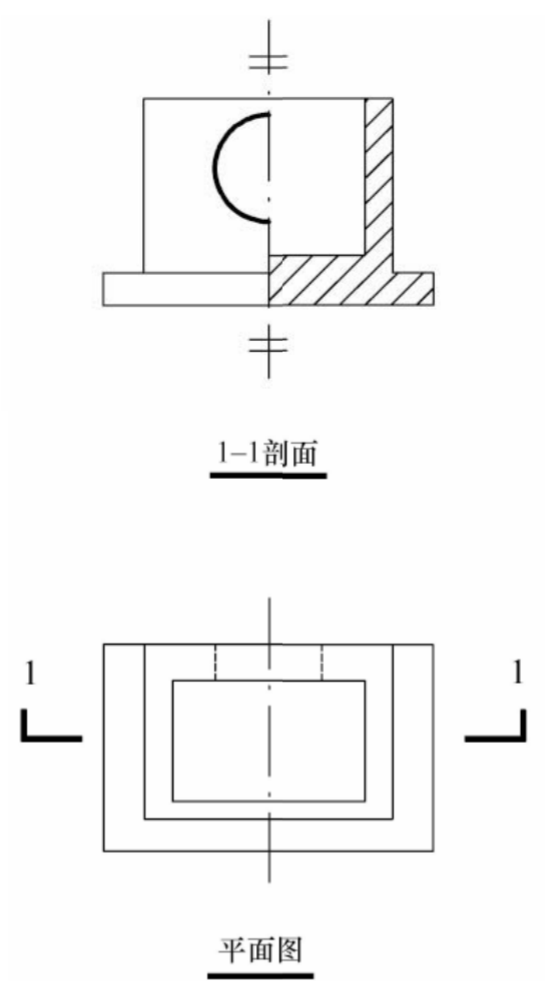
图 10.4.1-3 一半画视图，一半画剖面图
