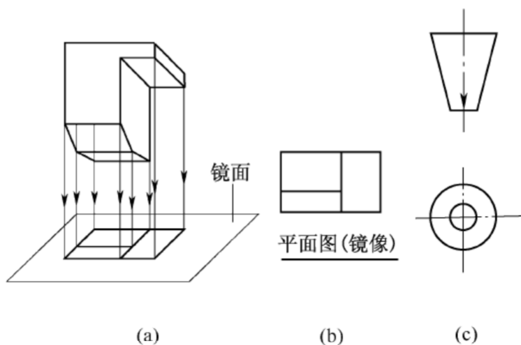
图 10.1.2 镜像投影法
