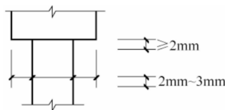
图 11.1.2 尺寸界线
