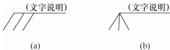
图 7.3.2 共用引出线
