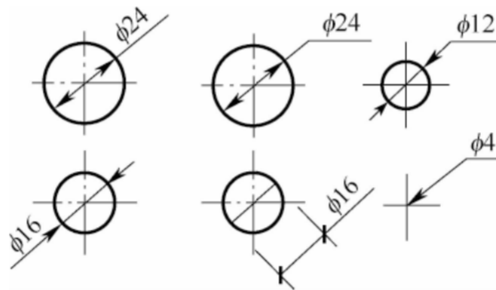
图 11.4.5 小圆直径的标注方法
