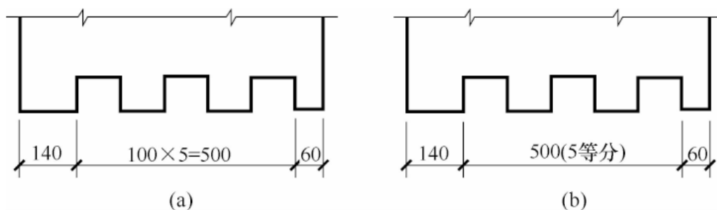
图 11.7.2 等长尺寸简化标注方法
