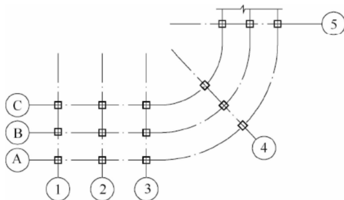
图 8.0.9-2 弧形平面定位轴线的编号
