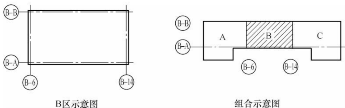
图 10.2.3 分区绘制建筑平面图
