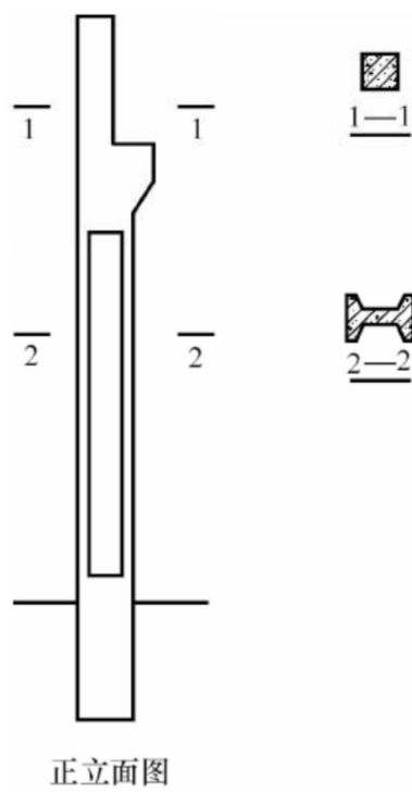
图 10.3.4-1 断面图按顺序排列
