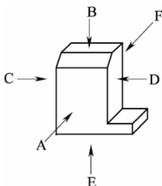
图 10.1.1 第一角画法
