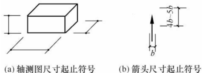
图 11.1.4 尺寸起止符号
