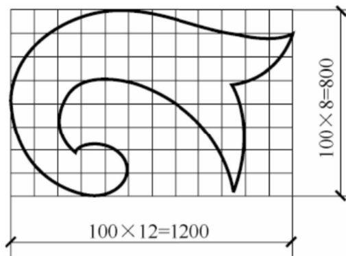
图 11.6.5 网格法标注曲线尺寸
