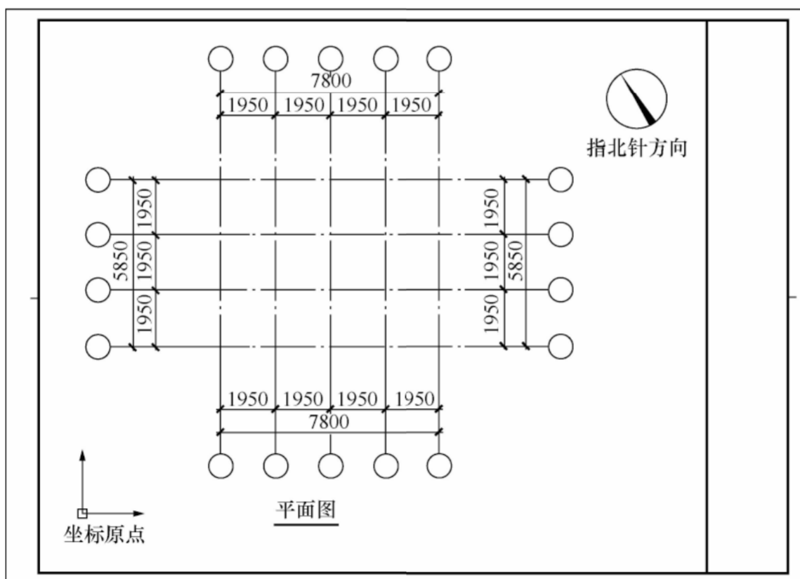
图 14.0.1-1 正交平面图制图方向与指北针方向示意
