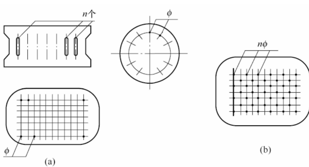
图 10.4.2 相同要素简化画法
