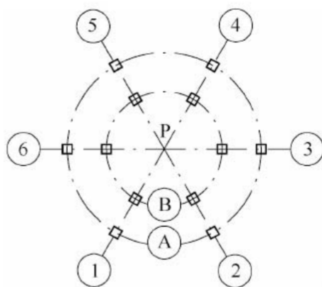
图 8.0.9-1 圆形平面定位轴线的编号
