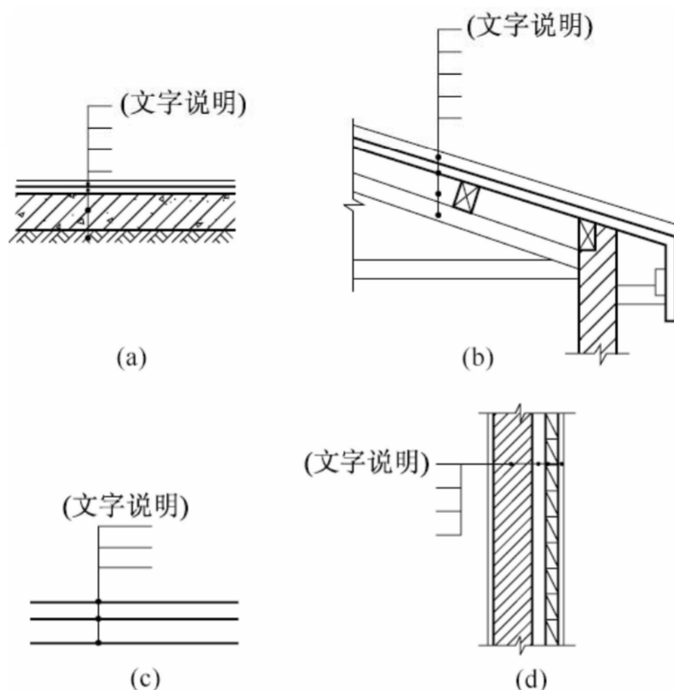
图 7.3.3 多层引出线
