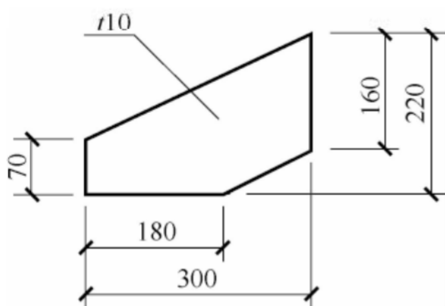
图 11.6.1 薄板厚度标注方法
