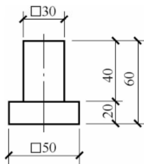
图 11.6.2 标注正方形尺寸
