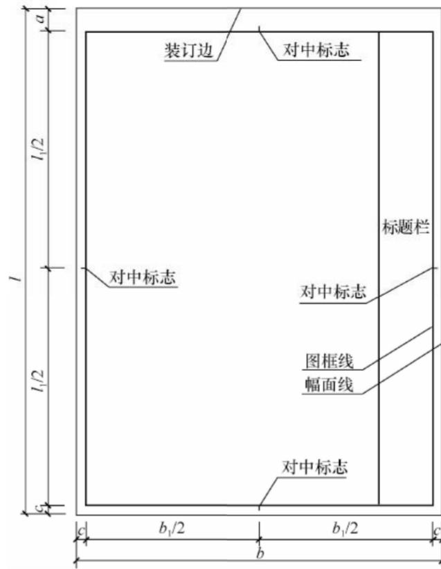
图 3.2.1-5 A0~A4 立式幅面 (二)
