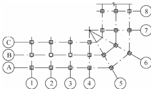
图 8.0.10 折线形平面定位轴线的编号
