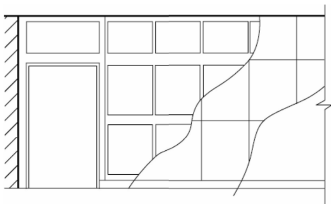
图 10.3.3 分层剖切的剖面图
