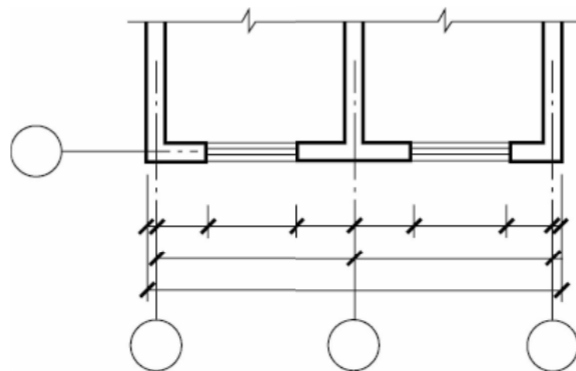
图 11.3.2 尺寸的排列
