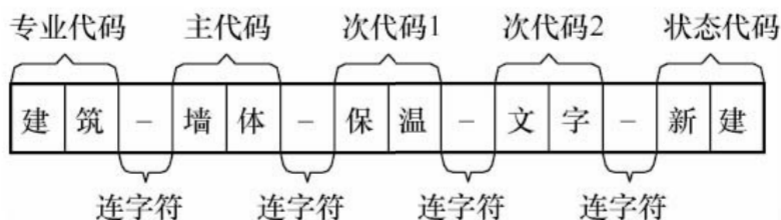
图 13.0.2-1 汉字图层命名格式
