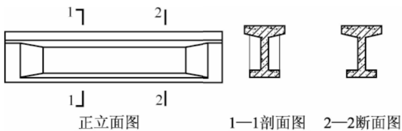
图 10.3.1 剖面图与断面图的区别
