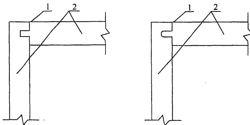
图 8.1.5-2 法兰垫料榫形接头密封示意
