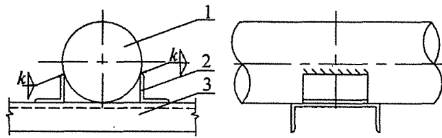
图 15 双侧挡板式固定支架示意
