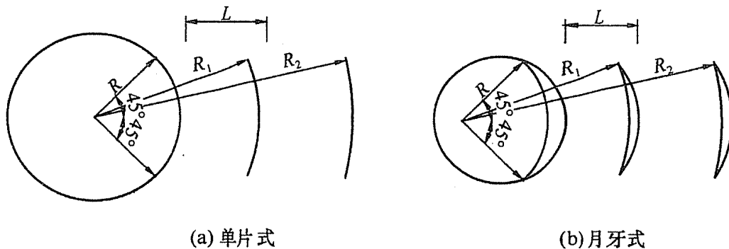
图 4.3.3 风管导流叶片形式示意
