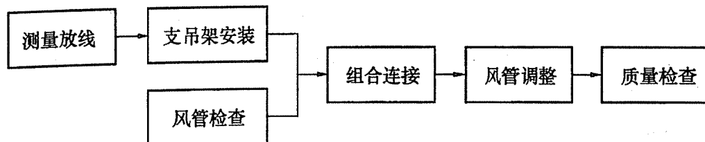
图 8.3.1 非金属与复合风管安装工序
