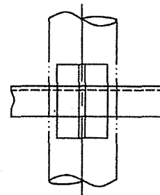
图 17 滑动支架示意
