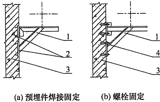
图 11 斜支撑型支架示意
