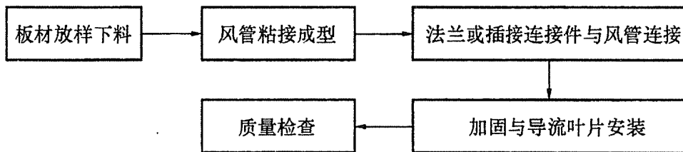
图 5.3.1 玻璃纤维复合风管与配件制作工序
