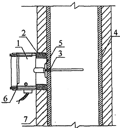
图 29 空气温度传感器的安装示意
