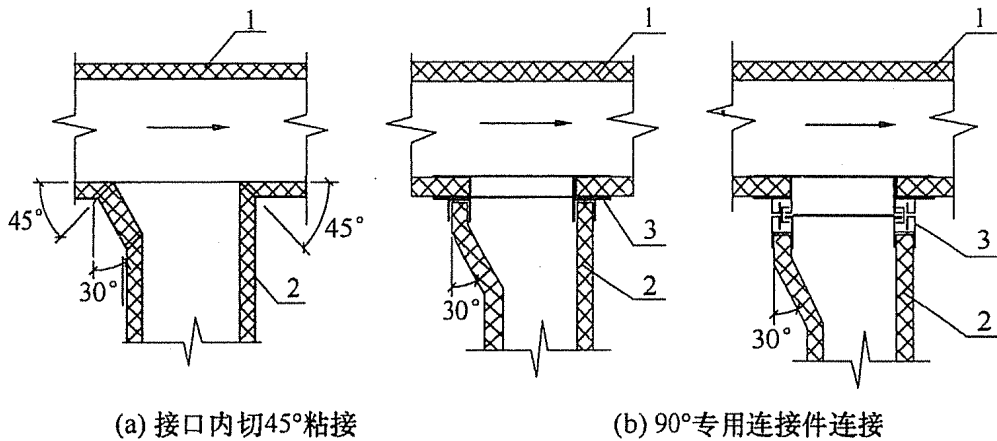
图 5.2.6 三通的制作示意
