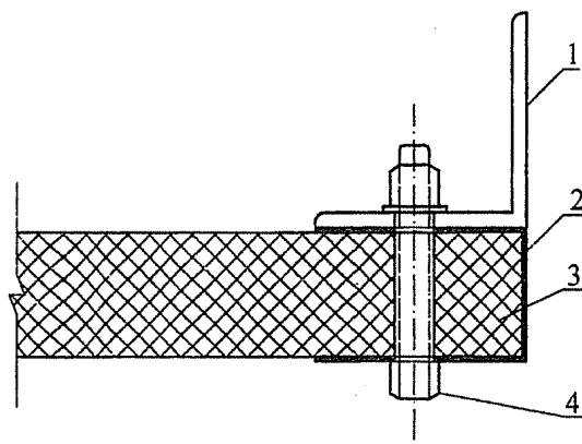
图 5.3.4 玻璃纤维复合风管角钢法兰连接示意
