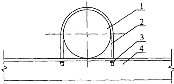
图 20 U 形管卡安装示意
