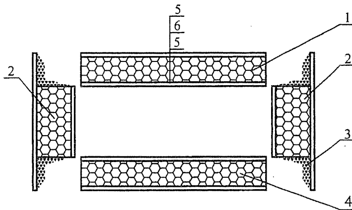
图 5.4.2-1 玻镁复合矩形风管组合示意
