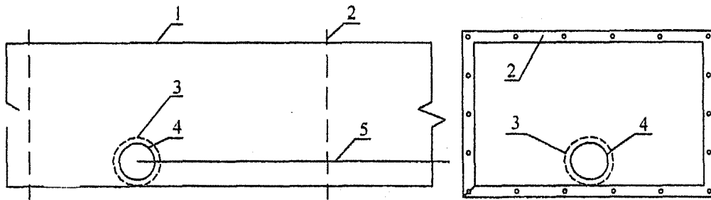
图 15.3.2 风管漏光检测示意
