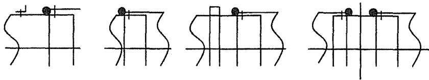
图 8.1.4-2 圆形风管连接的密封示意
