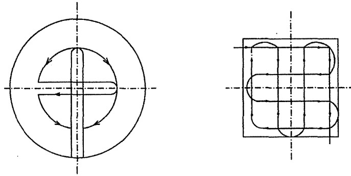
图 31 匀速移动测量路线
