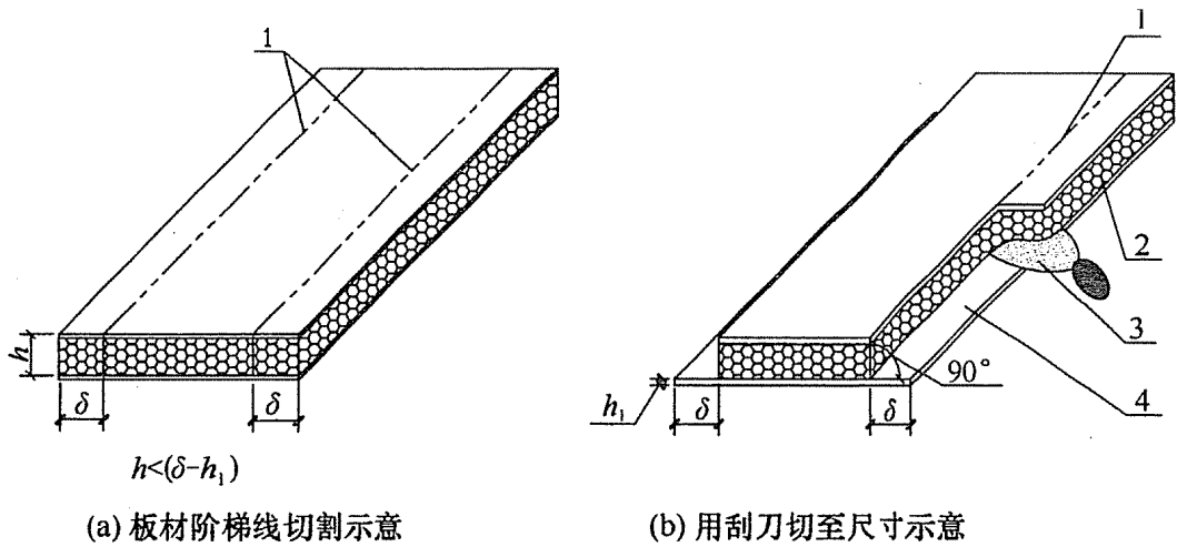
图 5.4.2-2 风管侧板阶梯线切割示意
