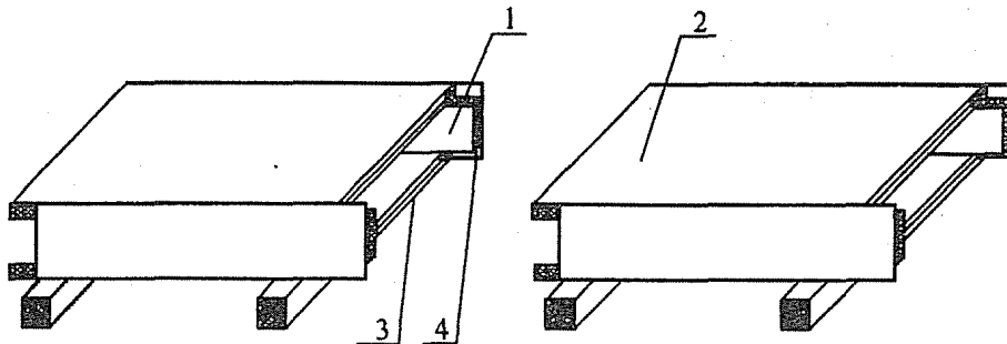
图 2 风管错位对口粘接示意
