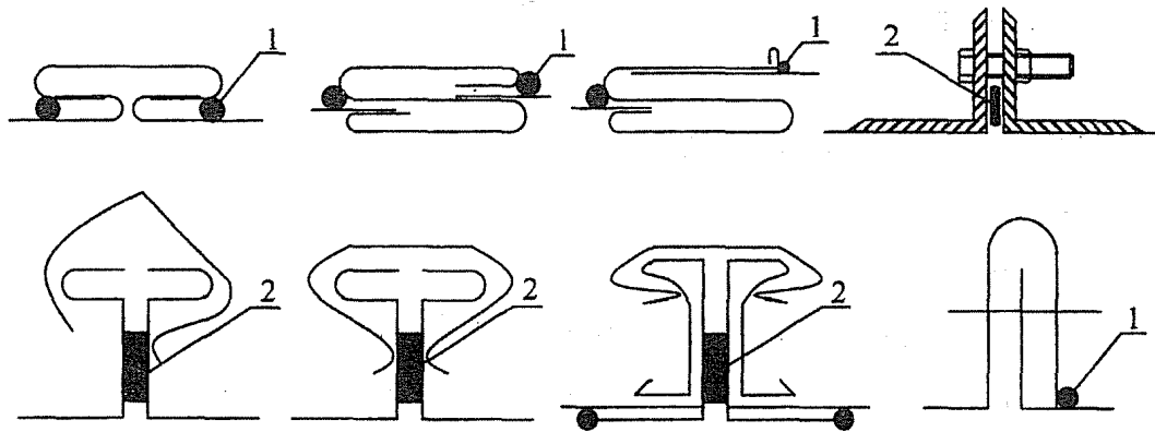
图 8.1.4-1 矩形风管连接的密封示意
