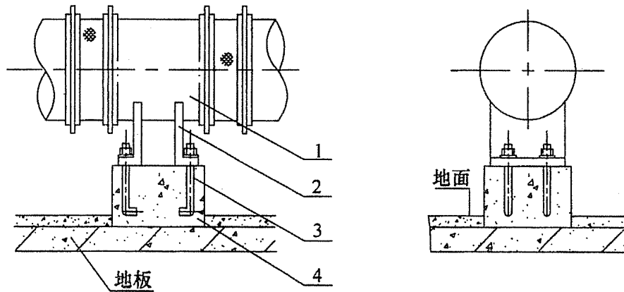
图 12 支撑型支架示意
