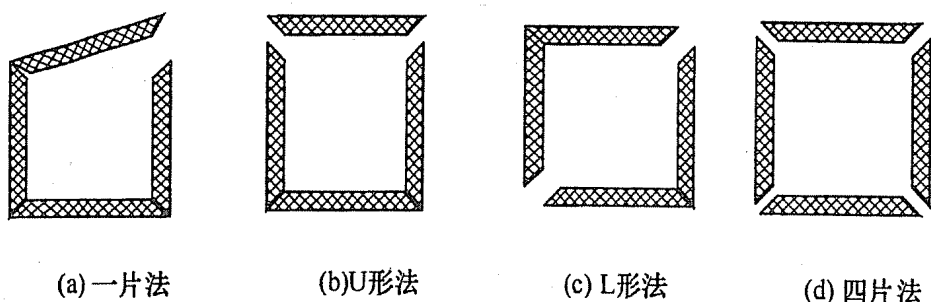
图 5.2.2-1 矩形风管 45°角组合方式示意
