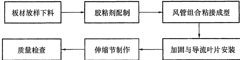
图 5.4.1 玻镁复合风管与配件制作
