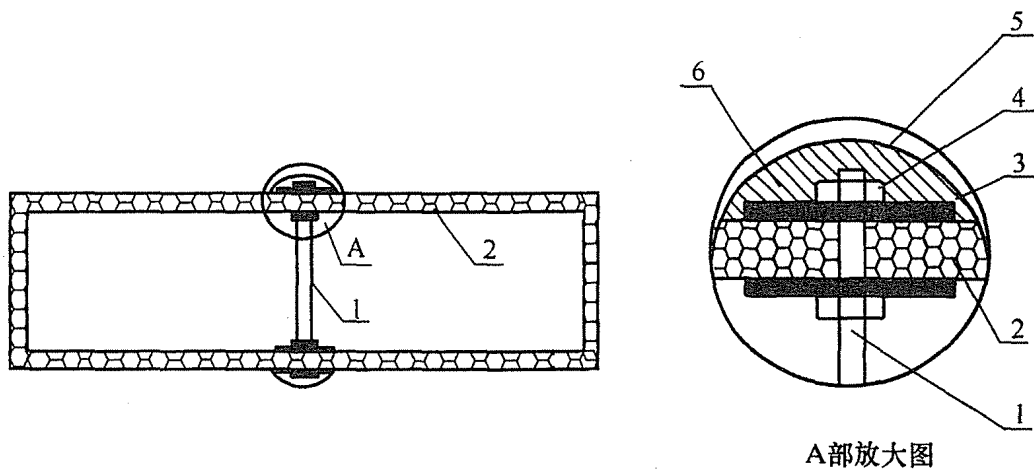
图 5.4.5 正压保温风管内支撑加固示意
