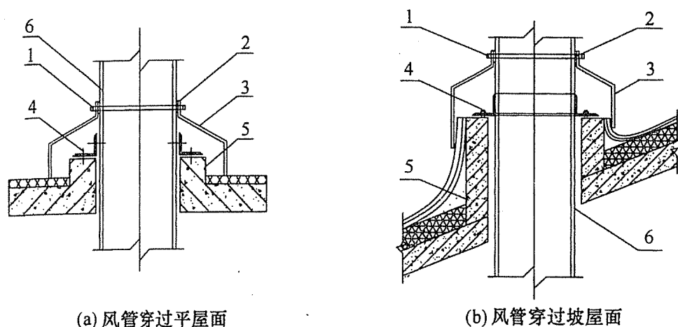
图 8.1.9 风管穿屋面防雨渗漏装置示意
