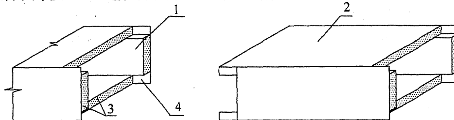
图 8.3.6-2 错位对接粘接示意
