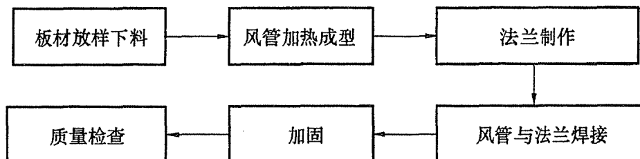
图 5.5.1 硬聚氯乙烯风管与配件制作工序
