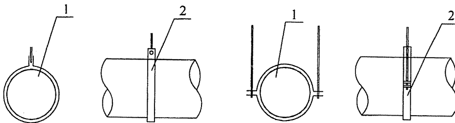
图 7.2.5-3 柔性风管吊环安装
