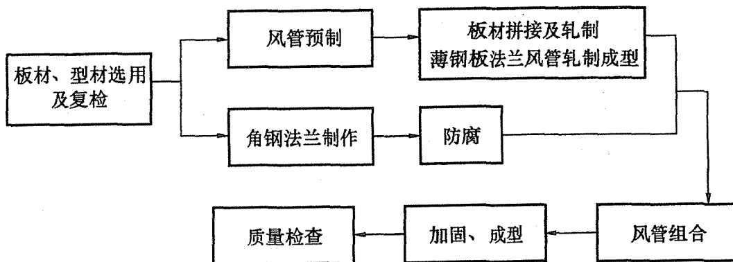
图 4.2.1 金属风管制作工序
