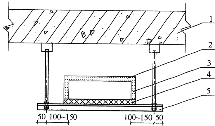
图 7.2.5-1 风管横担预留长度示意
