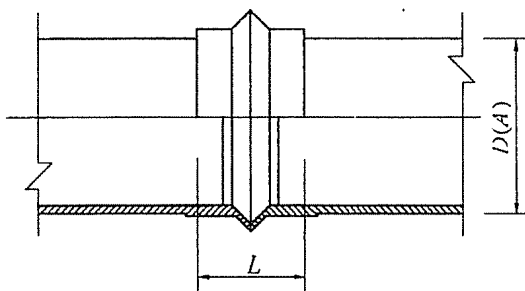
图 5.5.7-1 伸缩节示意
