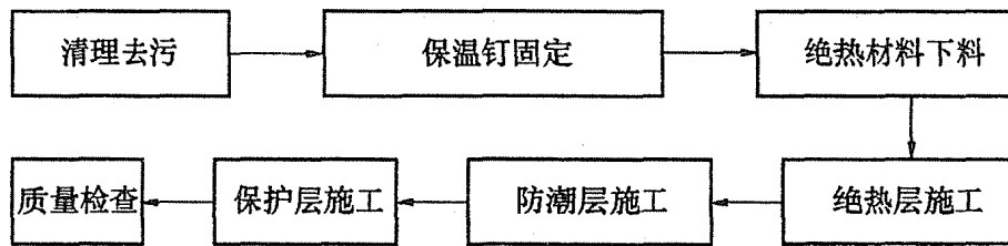
图 13.4.2 空调风管系统与设备绝热施工工序
