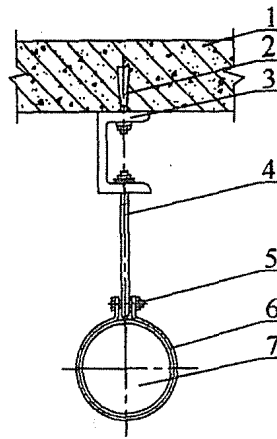
图 21 吊环安装示意
