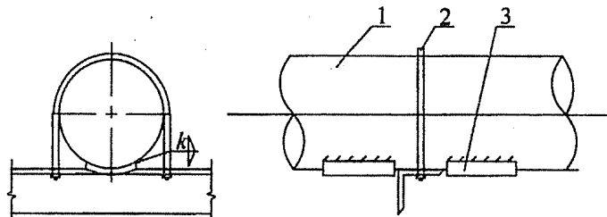
图 14 带弧形挡板管卡式固定支架示意
