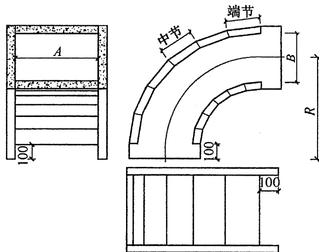
图 5.4.2-3 90°弯头放样下料示意
