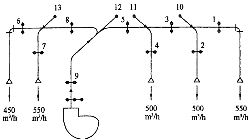
图 34 送风系统
