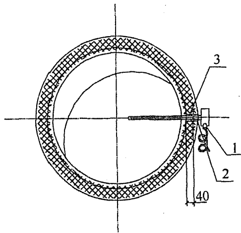
图 30 液体温度传感器安装图
