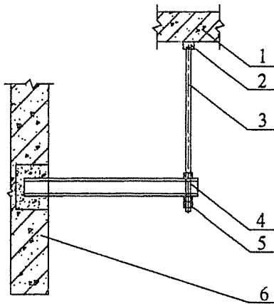
图 13 支架一端固定 一端悬吊安装示意
