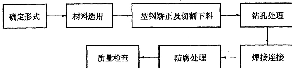
图 7.2.2 支、吊架制作工序
