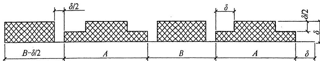
图 5.3.2-1 玻璃纤维复合风管 90°梯形槽口示意
