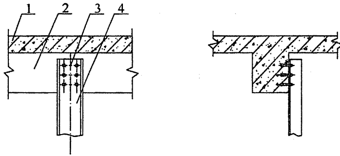
图 9 支架与梁固定示意
