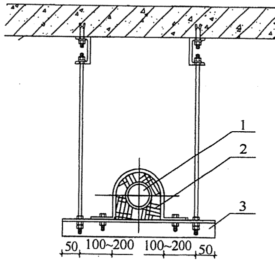
图 7.2.5-2 水管横担预留长度示意
