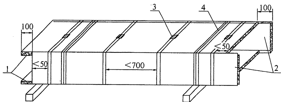
图 5.4.4-2 风管捆扎示意
