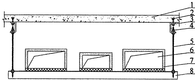
图 22 水平布置多风管共用吊架示意
