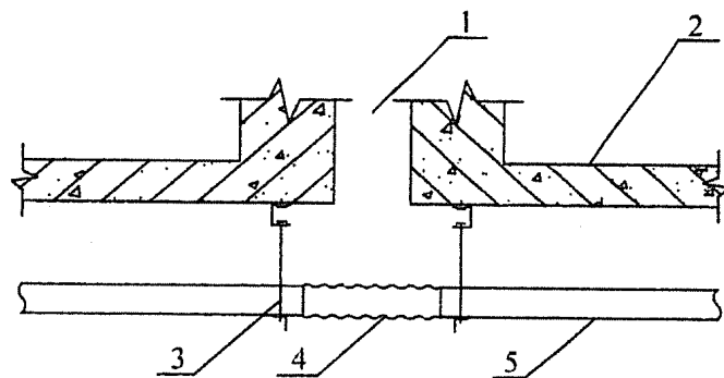
图 11.1.4-1 水管过结构变形缝空间安装示意
