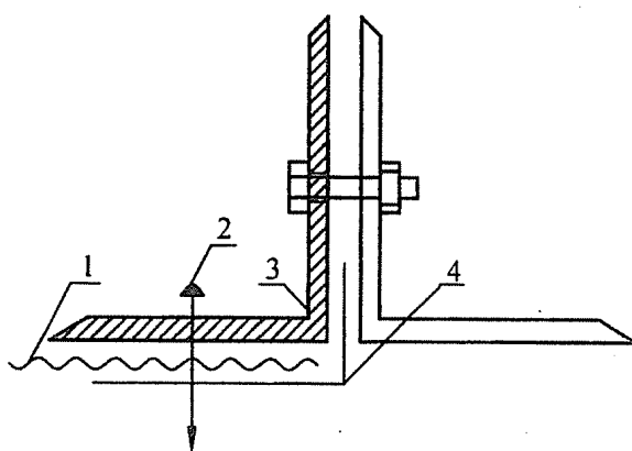
图6.6.3 柔性短管与角钢法兰连接示意
