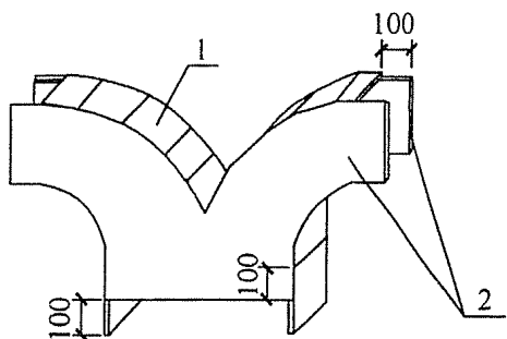
图 5.4.2-4 蝴蝶三通放样下料示意 1—外弧拼接板；2—平面板
