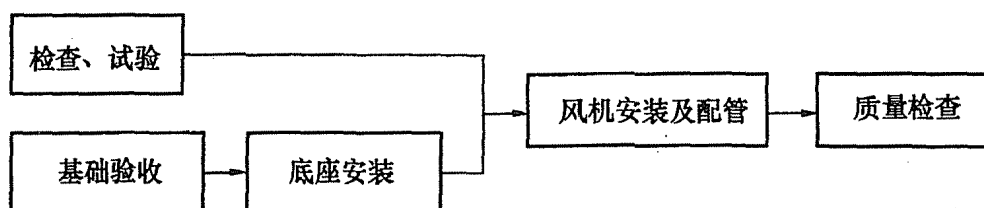
图 9.3.1 风机安装工序
