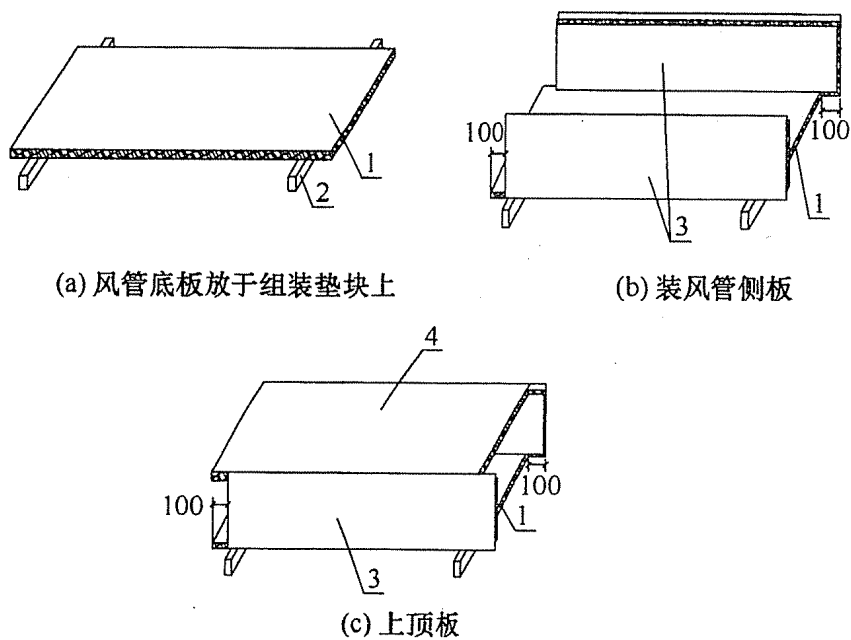
图 5.4.4-1 风管组装示意
