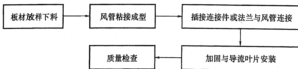
图 5.2.1 聚氨酯铝箔与酚醛铝箔复合风管及配件制作工序
