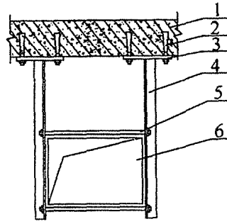
图 19 风管防晃支架示意
