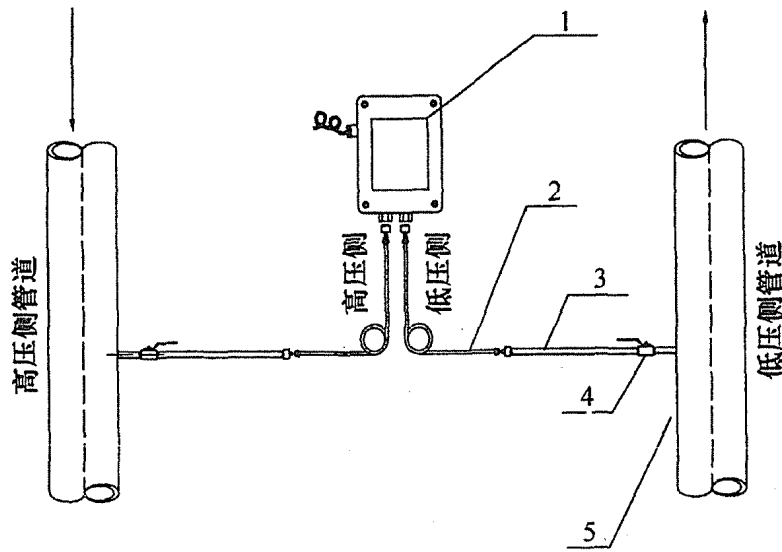
图 28 液体压差传感器（压差开关）安装示意
