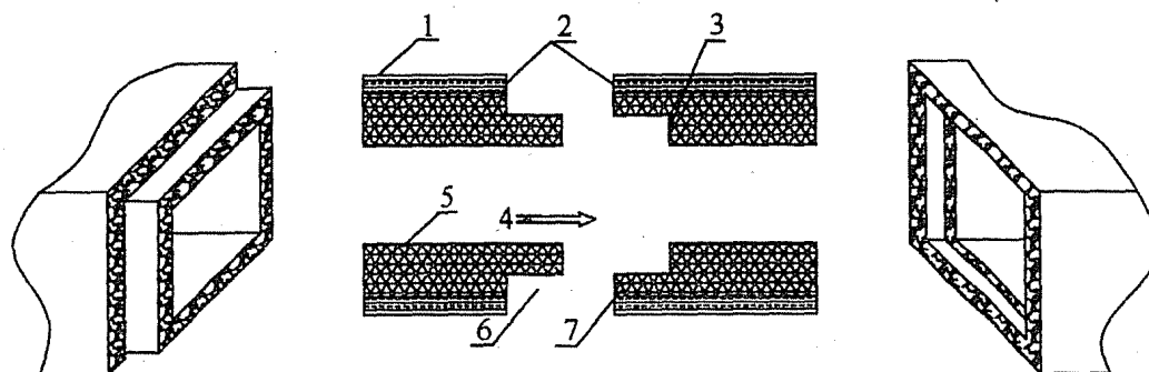
图 8.3.6-1 承插阶梯粘接接口示意
