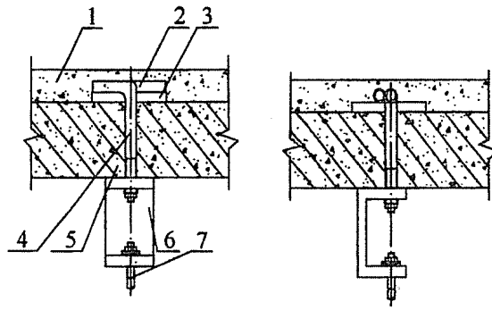
图 8 穿楼板螺栓固定示意
