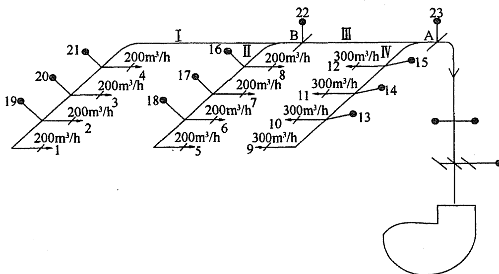
图 35 送风系统图
