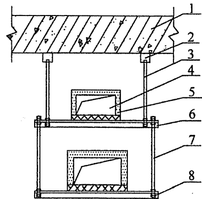
图 23 垂直布置双风管吊架示意
