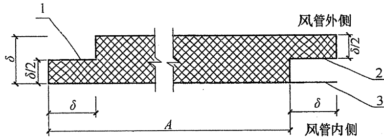
图 5.3.2-3 风管承插阶梯粘接示意
