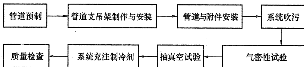
图 12.2.1 空调制冷剂管道与附件安装工序
