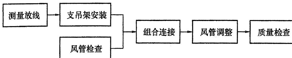
图 8.2.1 金属风管安装工序
