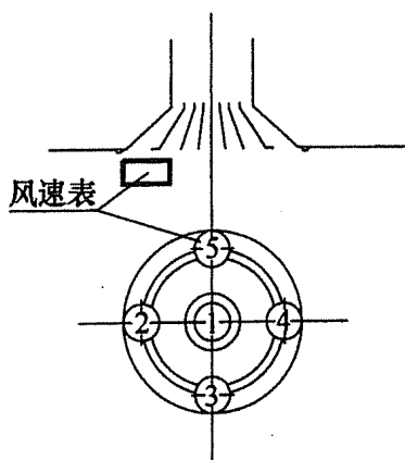
图 33 用风速仪测定散流器出口平均风速
