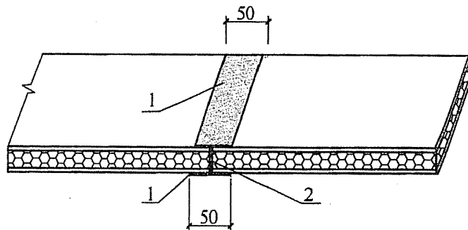
图 5.4.2-5 复合板拼接方法示意 1—玻璃纤维布；2—风管板对接处
