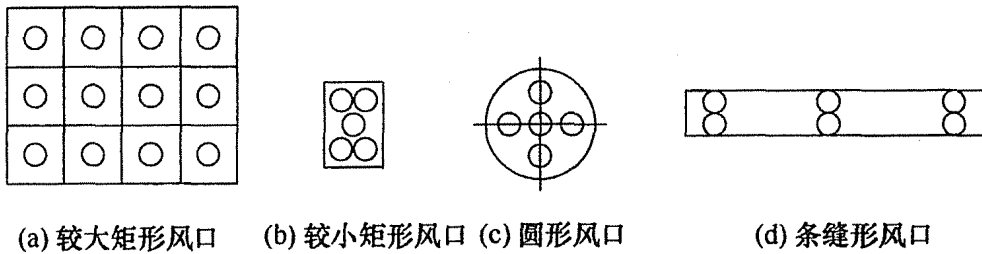
图 32 各种形式风口的测点布置示意
