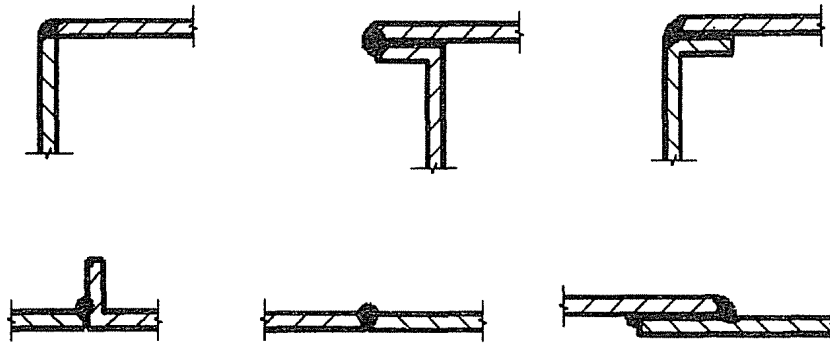
图 1 风管焊接焊缝形式示意
