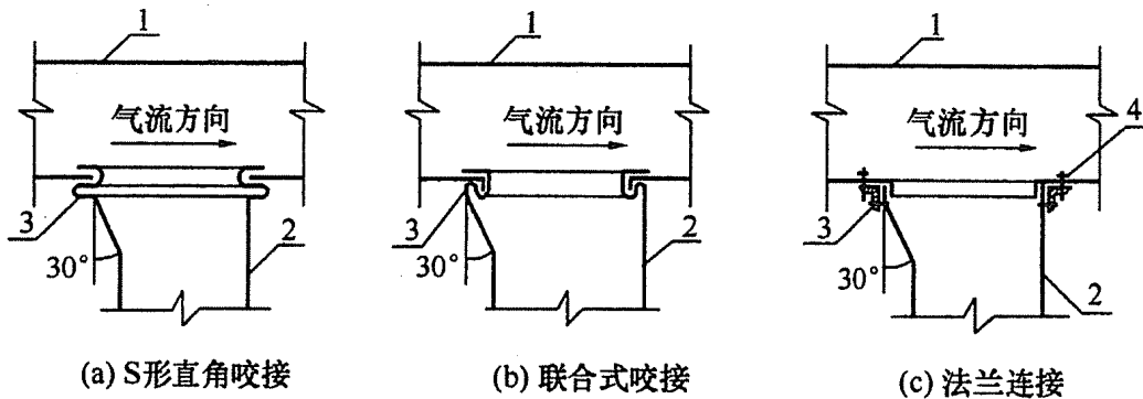
图 8.2.7 支风管与主风管连接方式
