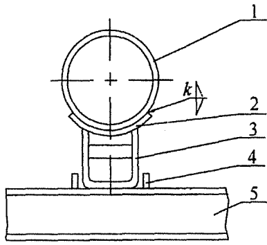
图 18 导向支架示意
