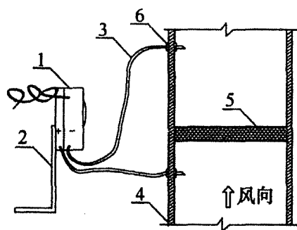
图 27 空气压差传感器
