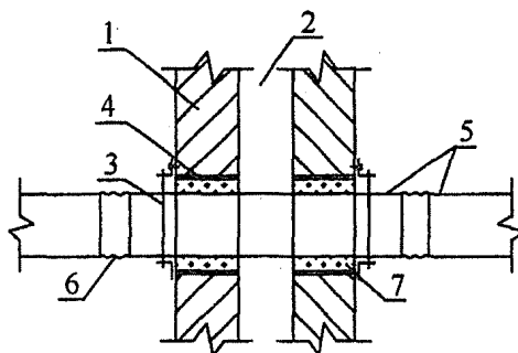
图 8.4.3-2 风管穿越变形缝墙体的安装示意
