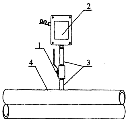
图 26 液体压力传感器安装示意
