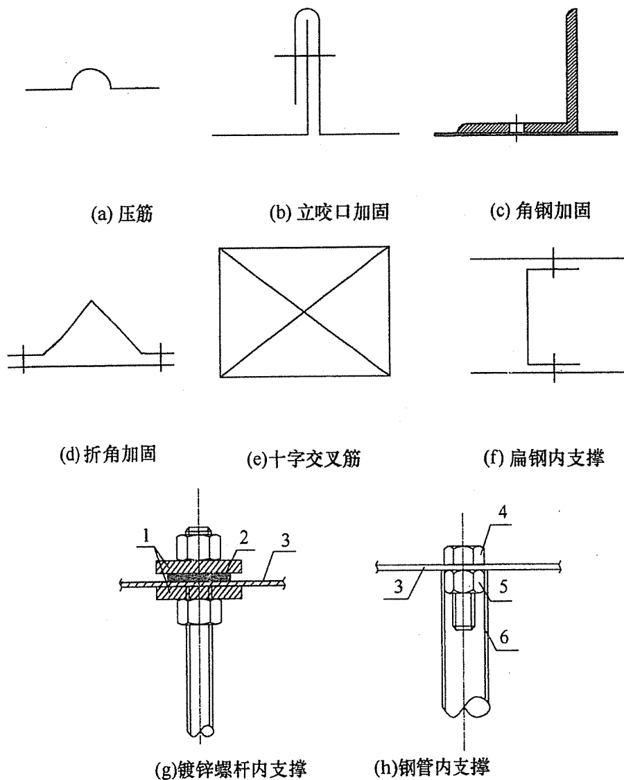
图 4.2.15 风管加固形式示意
