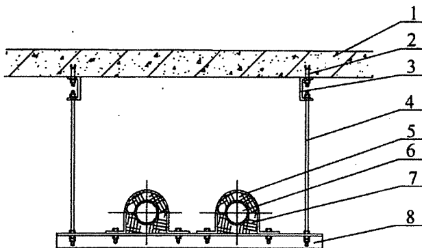
图 24 水管双管道共用悬吊架示意
