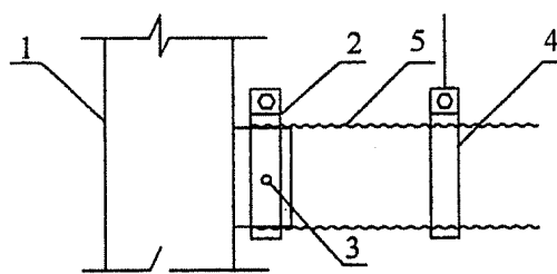
图 8.4.4 卡箍（抱箍）连接示意 1—主风管；2—卡箍；3—自攻螺钉； 4—抱箍吊架；5—柔性风管
