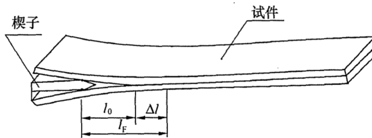
图 C.6.1 裂缝开展示意图
