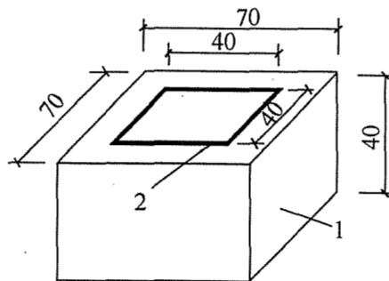
图 G. 3. 1-1 混凝土试块形式及尺寸 (mm)
