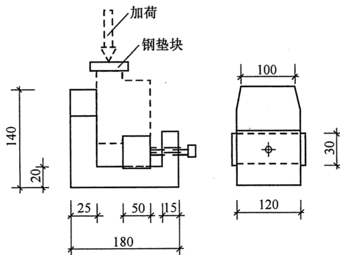
图 N.2.2 剪切加荷装置构造示意图 (mm)
