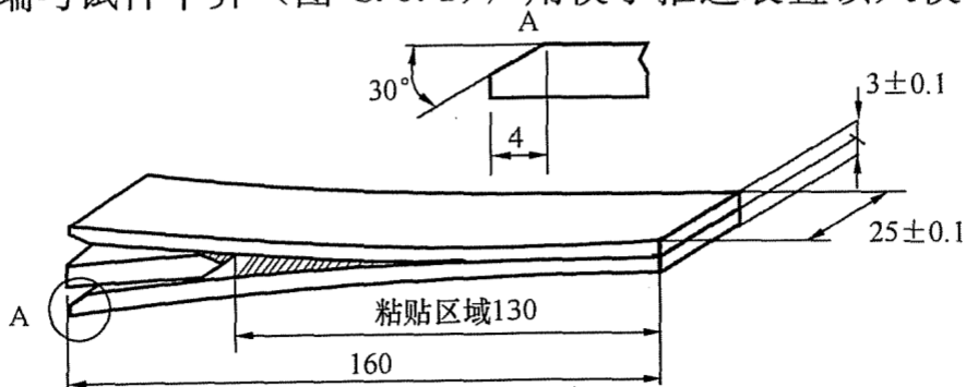
图 C. 5. 1 试件与楔块示意图 (mm)
