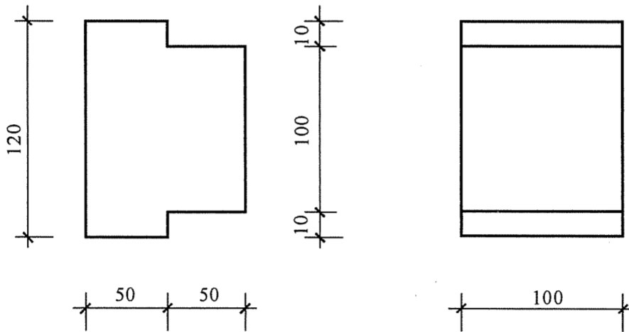
图 N.3.1 混凝土凸形块 (mm)
