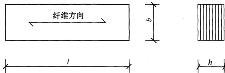
图 D.4.2 试件形状及尺寸符号
