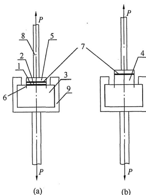
图 G.3.5 试件组装
