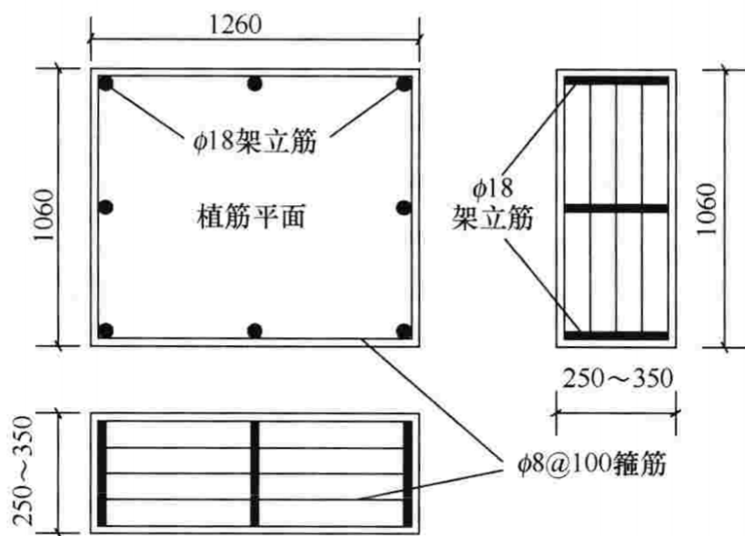
图 K. 2.3 植筋用混凝土块体配筋图
