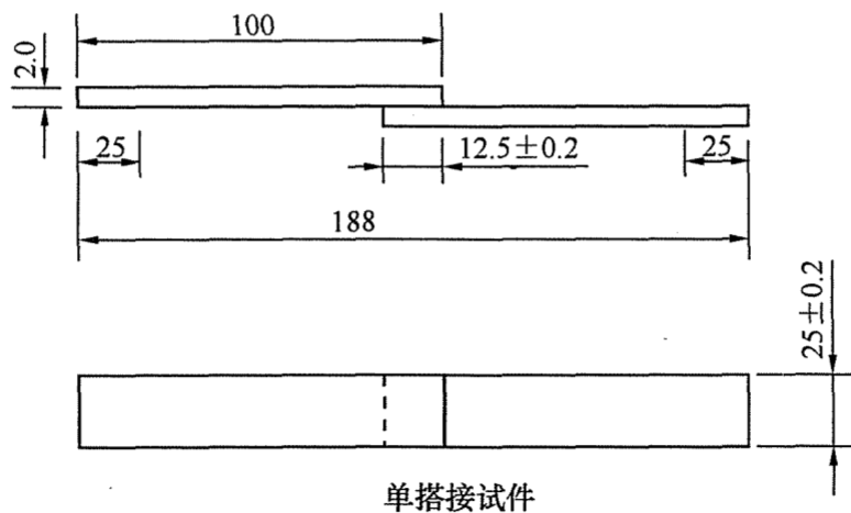
图 M.3.1-1 试件形状和尺寸 (一) (mm)
