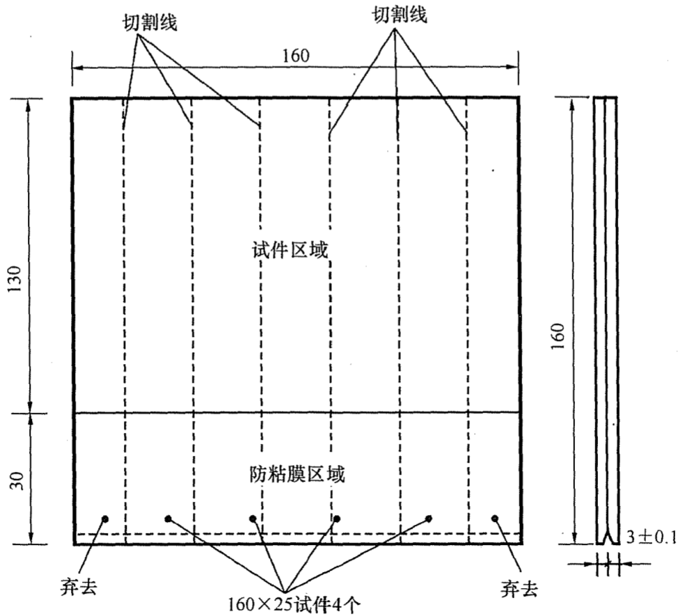
图 C. 4. 1 试板形式和尺寸 (mm)
