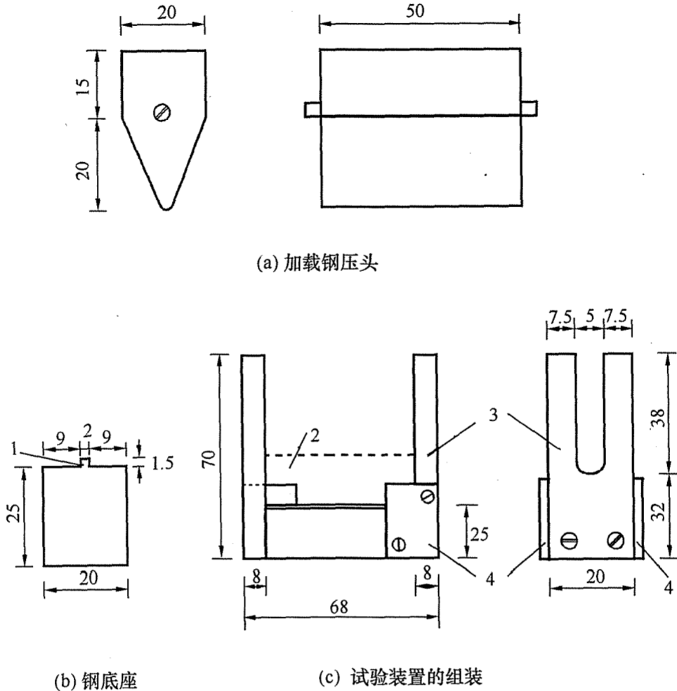
图 E.3.3 劈拉试验装置 (mm)
