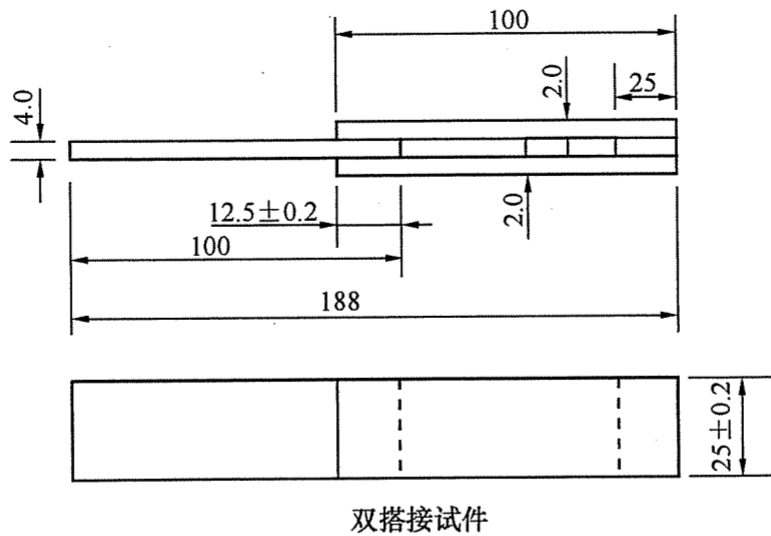
图 M. 3. 1-2 试件形状和尺寸 (二) (mm)
