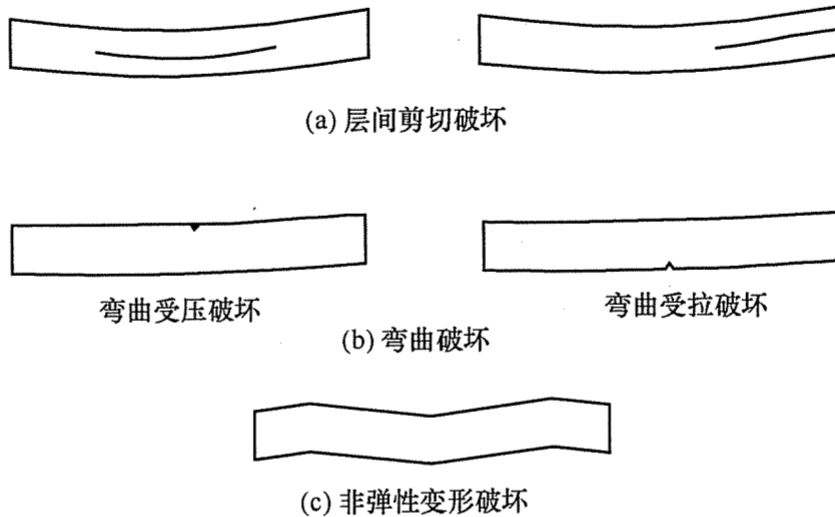
图 D. 7. 2 试件的破坏形式
