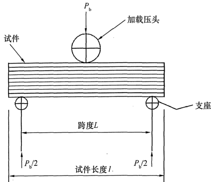
图 D.5.2 试验装置示意图
