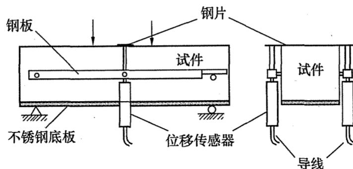
图 T.2.4 弯曲试验挠度测量示意图
