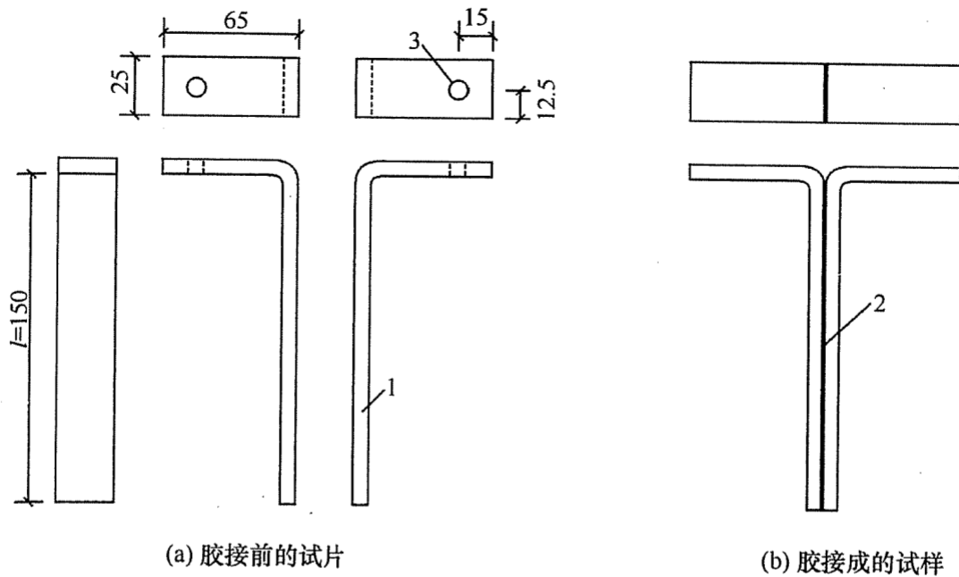
图 F. 4. 1 T 冲击剥离试样尺寸 (mm)
