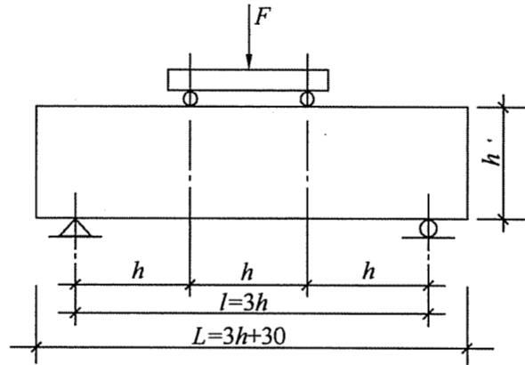
图 S. 2.5 抗折试验装置 (mm)
