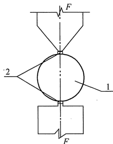
图 E. 4. 1 试件安装示意图 1—试件；2—木垫条
