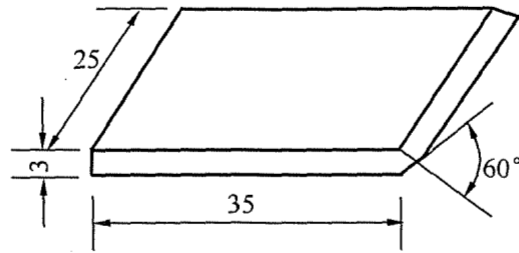
图 C. 3. 2 楔子试件形式及尺寸 (mm)
