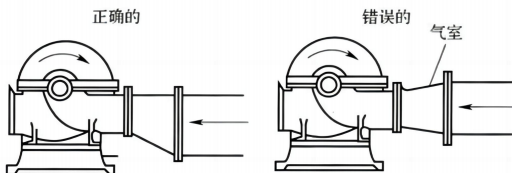
图1 正确和错误的水泵吸水管安装示意图
