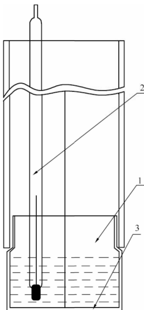
图 E.0.1 露点仪
