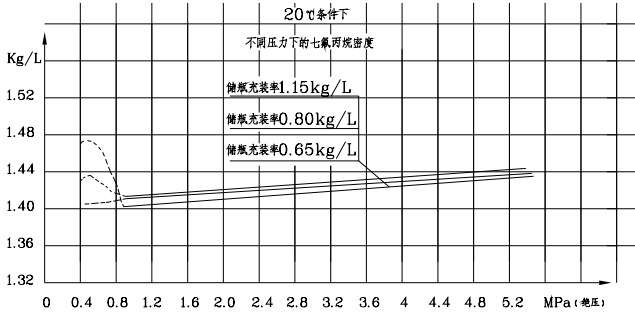
图 3.3.15-2 不同压力下七氟丙烷的密度
