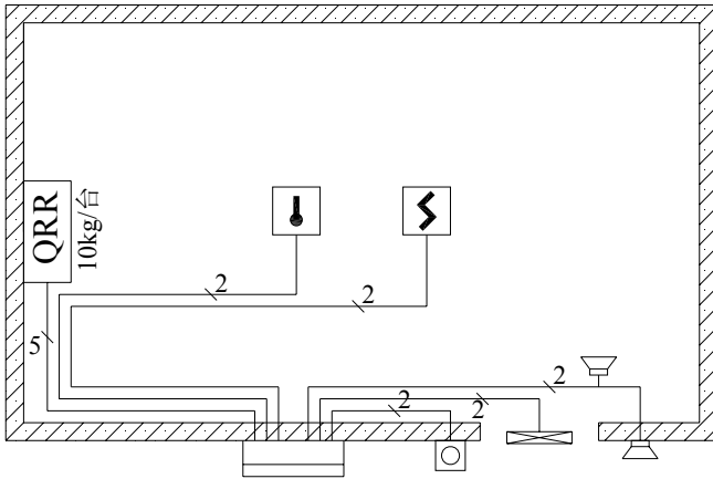
图例： 热气溶胶灭火装置 连线数 灭火控制器 喷放指示灯 感温探测器 紧急启动按钮 感烟探测器 声光报警器
