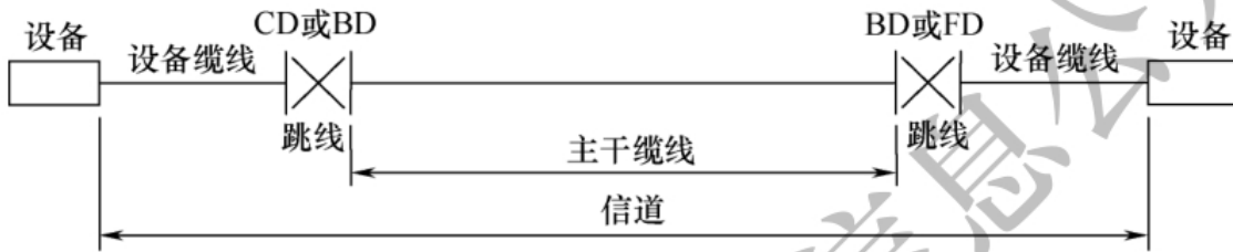
图 3.3.3-2 干线子系统信道连接方式
