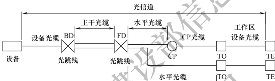
图 3.2.4-1 光纤信道构成 1
