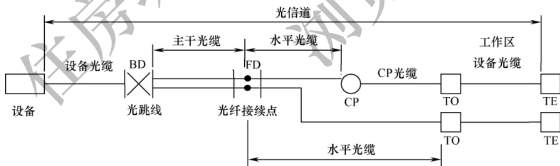
图 3.2.4-2 光纤信道构成 2
