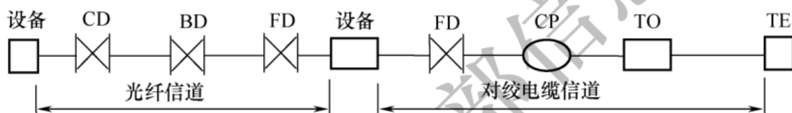
图 3.1.2-4 综合布线系统应用典型连接与组成
