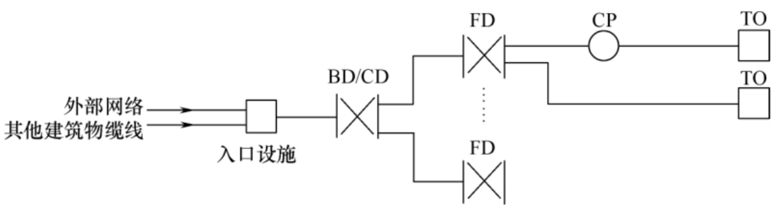
图 3.1.2-3 综合布线系统引入部分构成
