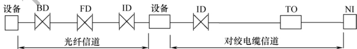
图 3.7.6 工业环境布线系统光纤信道与电缆信道构成
