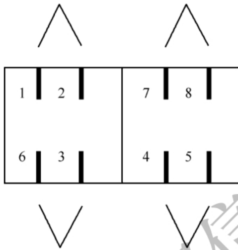
图 6.1.3-3 7类和7 A 类插座连接(正视)方式2
