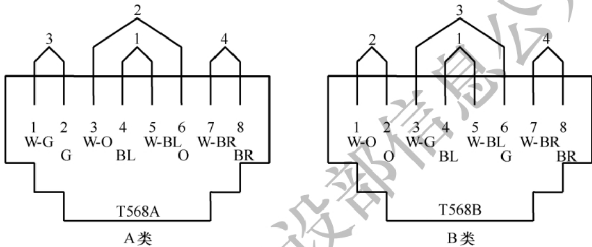
图 6.1.3-1 8 位模块式通用插座连接
