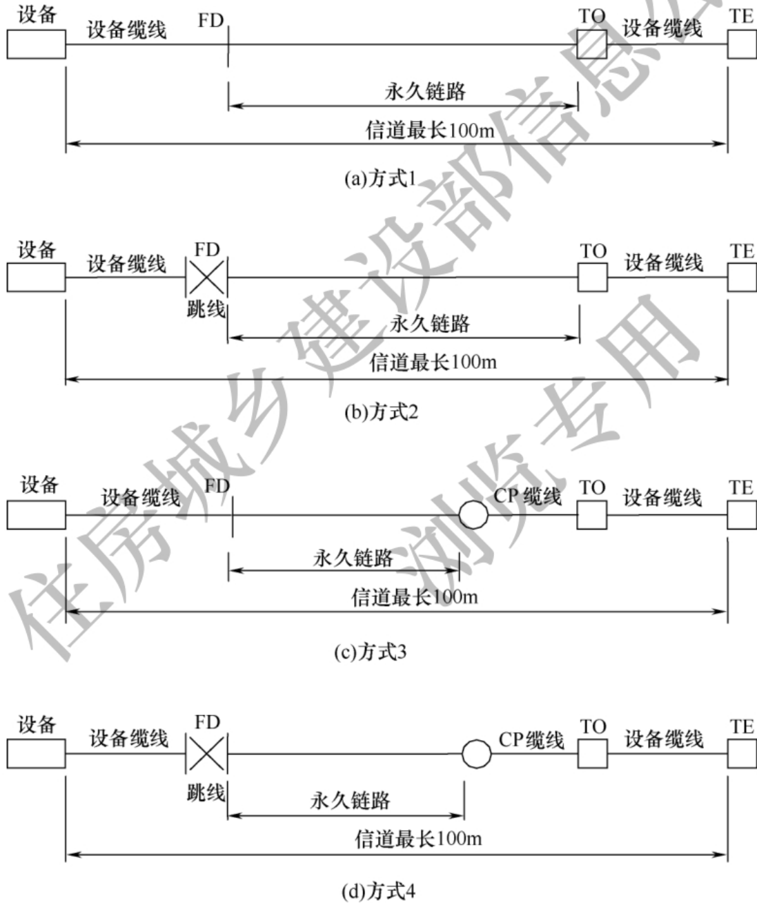
图 3.3.3-1 配线子系统信道连接方式
