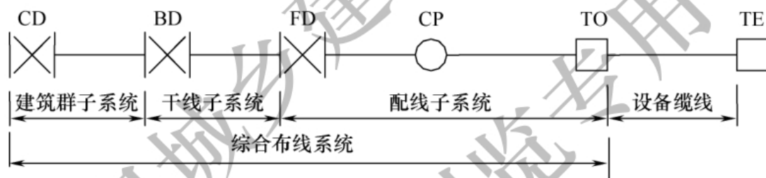
图 3.1.2-1 综合布线系统基本构成
