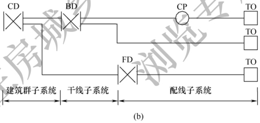
图 3.1.2-2 综合布线子系统构成
