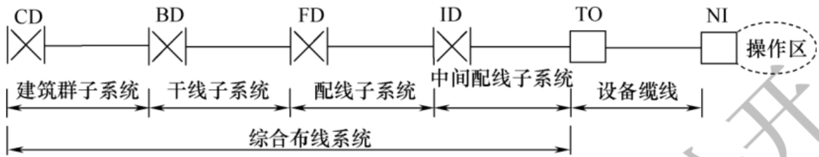
图 3.7.3 工业环境布线系统架构
