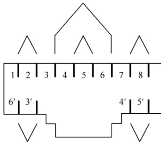
图 6.1.3-2 7 类和 7 A 类模块插座连接(正视)方式 1
