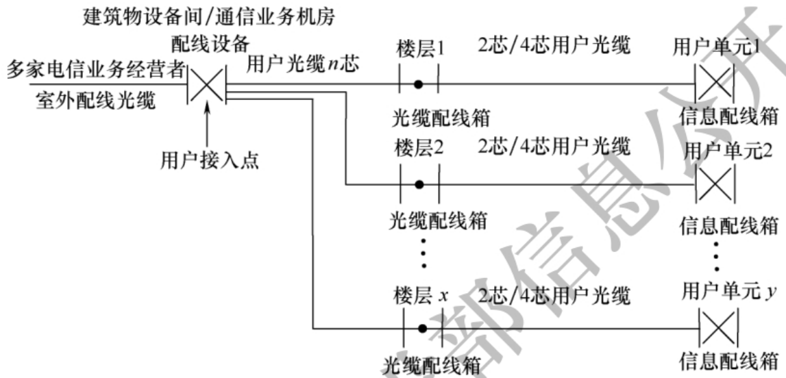
图 4.2.2-1 用户接入点设于独栋建筑物内设备间
