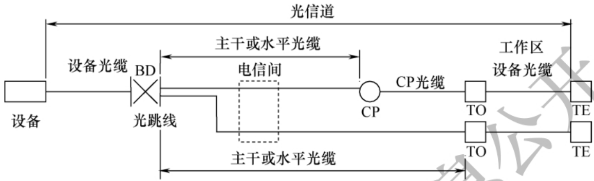
图 3.2.4-3 光纤信道构成 3
