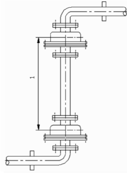
图 7.11.5—2 球形补偿器球心距的安装长度
