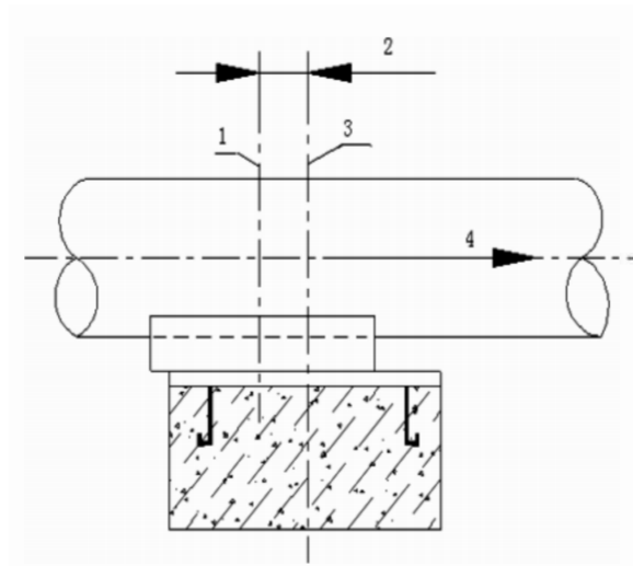
图 7.12.5 滑动支架安装位置
