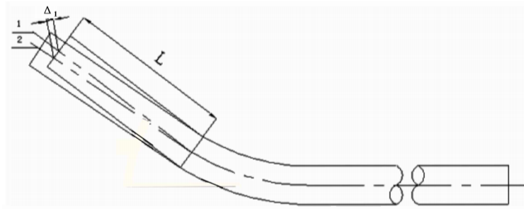
图 5.3.7-2 弯管的管端中心偏差
