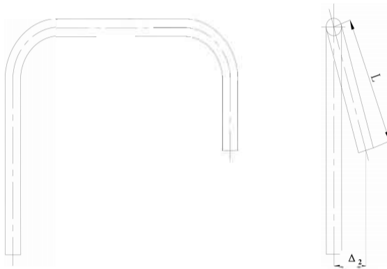
图 5.3.8 II 形弯管平面度
