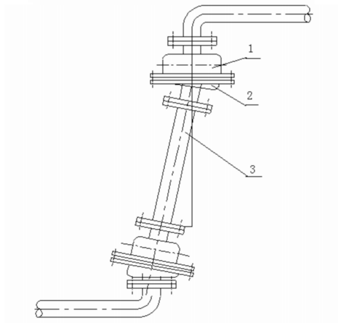
图 7.11.5—1 球形补偿器与球心距管段的组合
