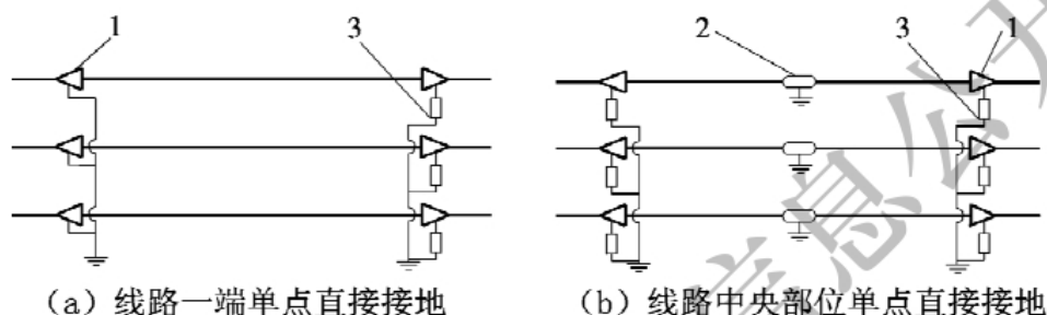
图 4.1.12-1 线路一端或中央部位单点直接接地
