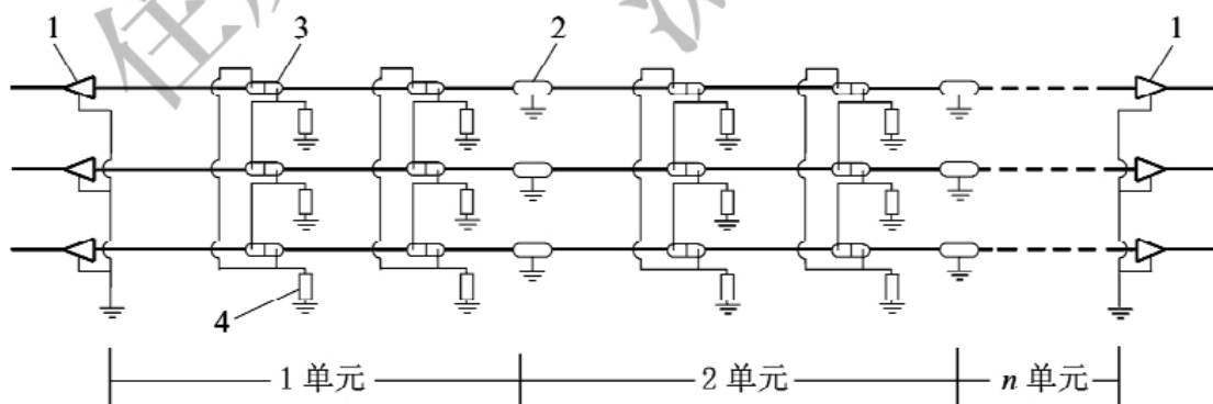
图 4.1.12-3 交叉互联接地
