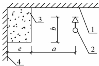
图 7.2.5 喷头与靠墙障碍物的距离
