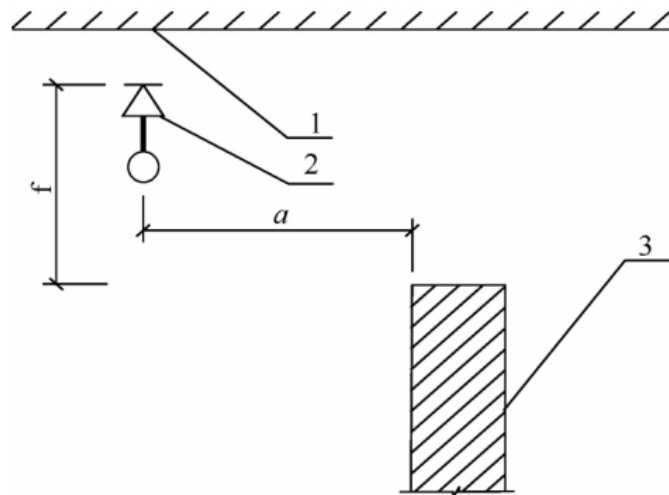
图 7.2.4 喷头与不到顶隔墙的水平距离
