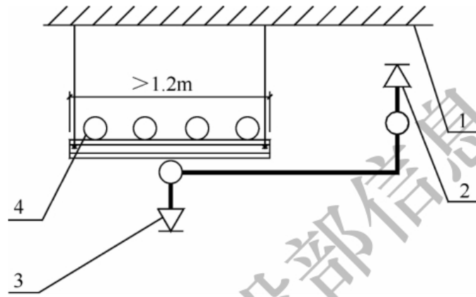
图 7.2.3 障碍物下方增设喷头
