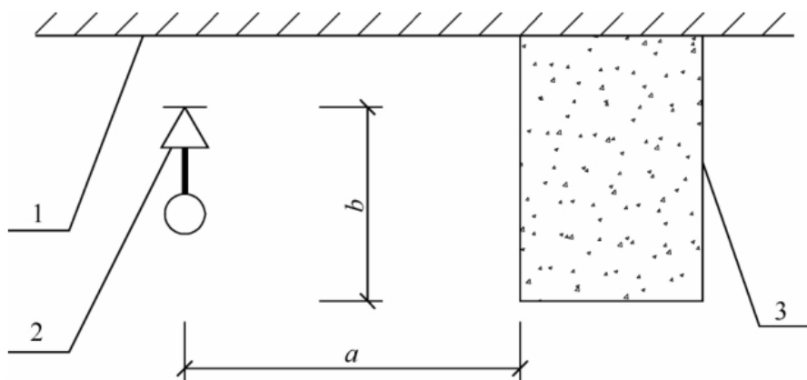
图 7.2.1 喷头与梁、通风管道等障碍物的距离
