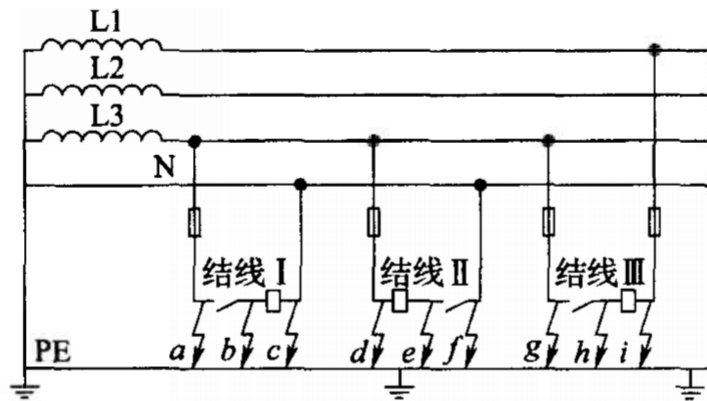
图 1 控制回路结线示例图
