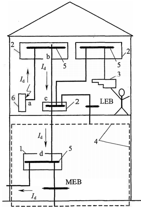
图 6 同一配电箱或配电干线间接引出的不同回路 1—进线配电箱；2—配电箱；3—手持式电气设备；4—结构钢筋； 5—保护导体；6—固定式电气设备
