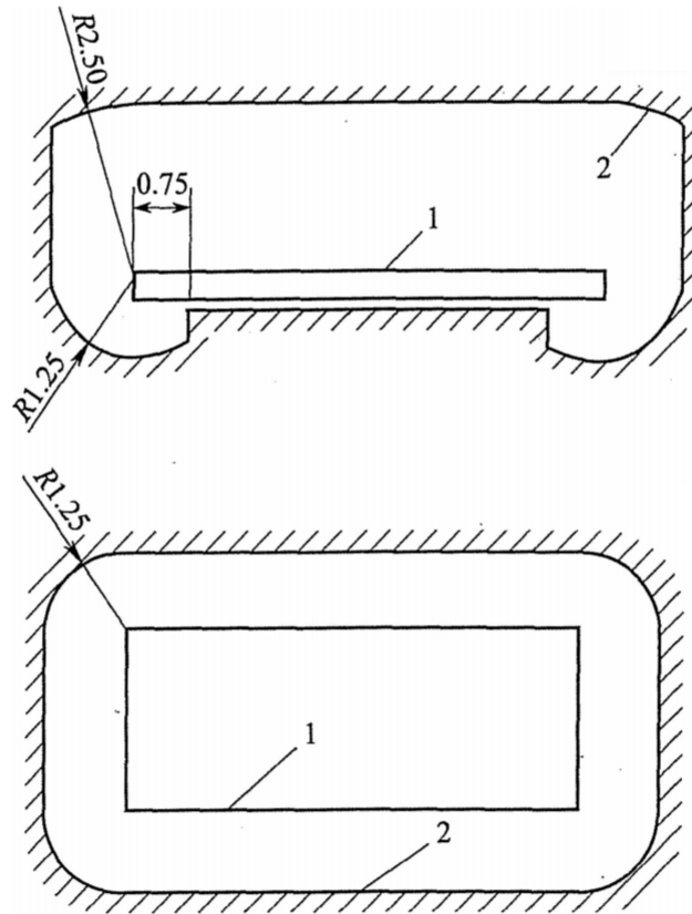
图 5.1.11 伸臂范围(m)
