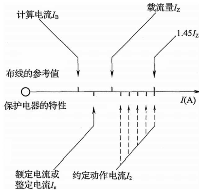
图 7 过电荷保护电器的动力特性关系图
