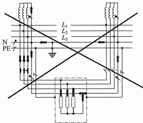
图 1 在 TN-S 系统中,产生杂散电流的例子
