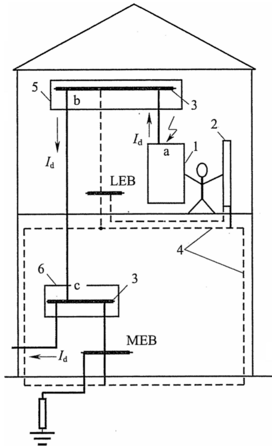
图3 局部等电位联结的作用
