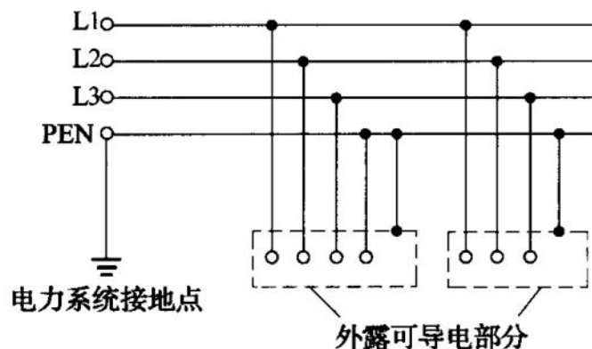
图 5 TN-C 系统
