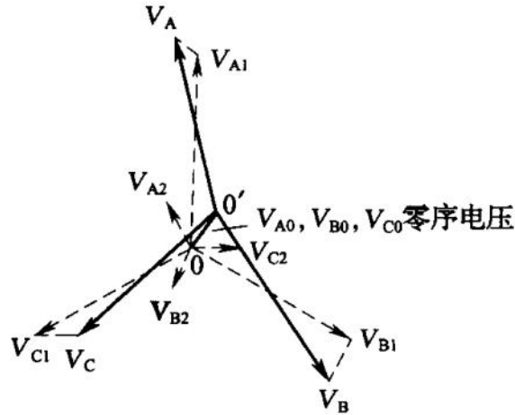
图 3 不对称电压向量图
