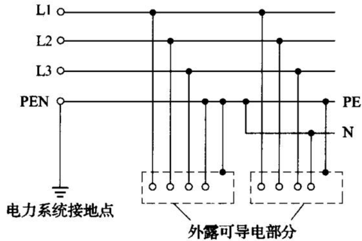
图 6 TN-C-S 系统
