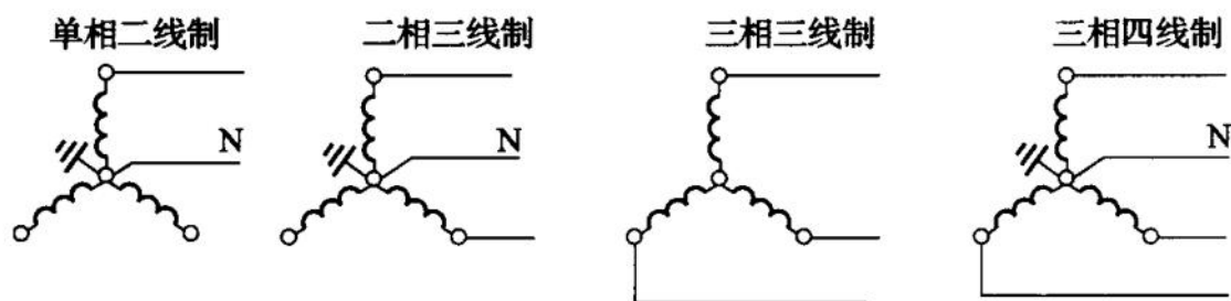
图 4 交流系统带电导体类型
