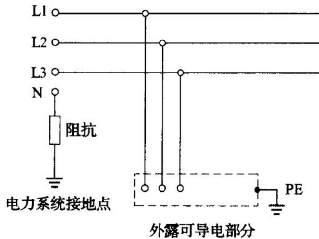
图 9 IT 系统
