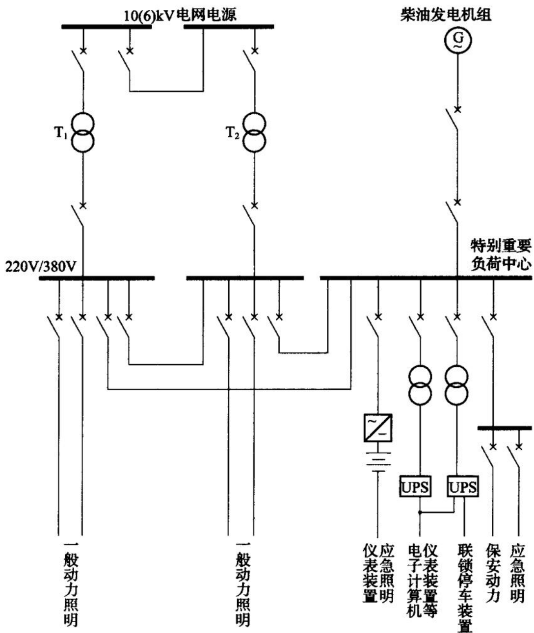
图 1 应急电源接线示例
