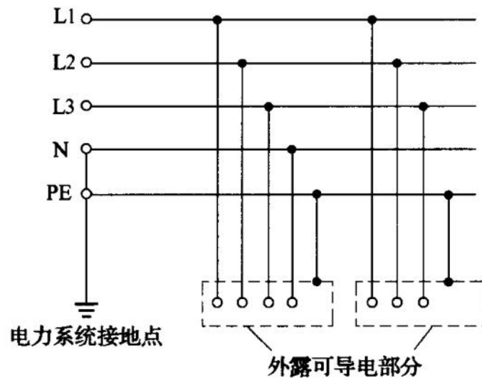
图 7 TN-S 系统
