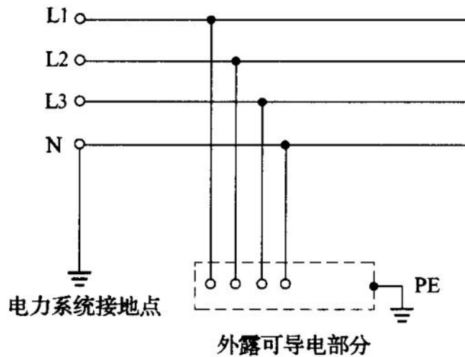
图 8 TT 系统
